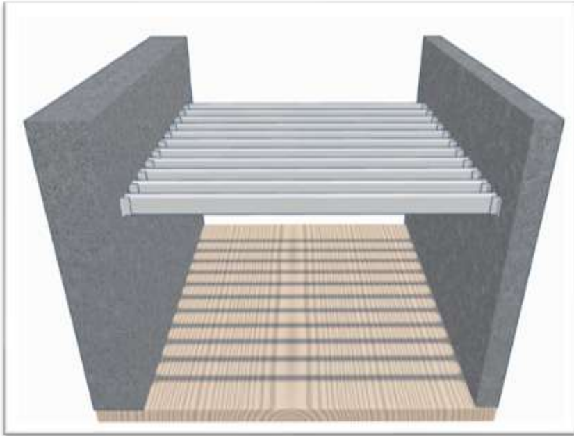
Doble Muro – Opción 5
