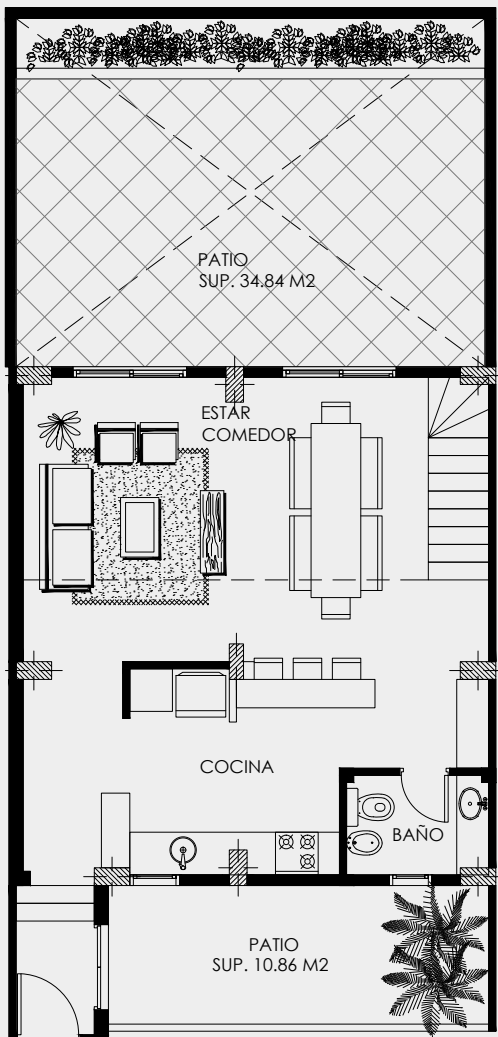
PLANTA BAJA
