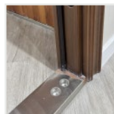
7 UMBRAL DE ACERO INOXIDABLE.
