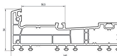
11290: Marco Evolution
