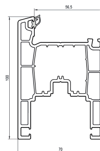
11090: Hoja Evolution
