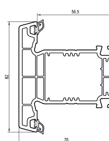
11127: Poste 70
