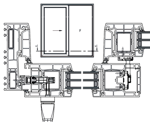
11290: Marco Evolution
