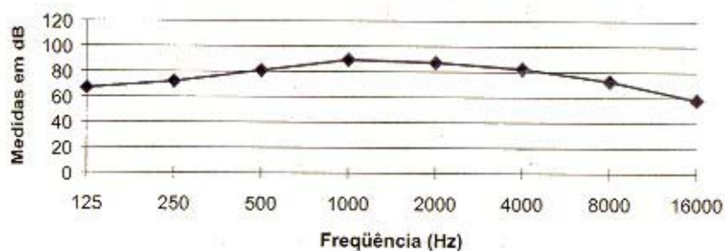
FIGURA 31 – Espectro sonoro de betoneira (1/4 da carga total)
