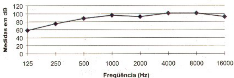
FIGURA 24 – Espectro sonoro de policorte ( corte de ferragens)
