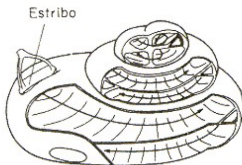
FIGURA 8 - A cóclea e os dutos FONTE - GERGES (1992), p. 45
