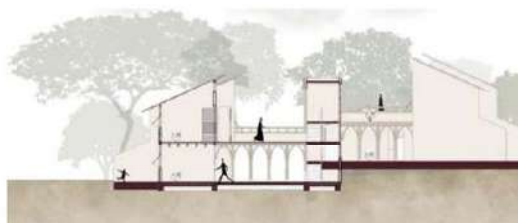
Corte A-A Vivienda II Etapa Final
