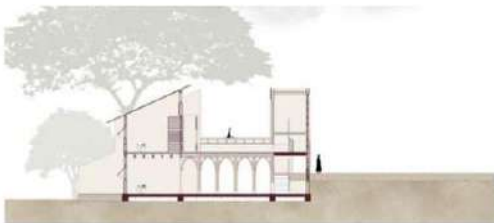
Corte A-A Vivienda I Etapa inicial
