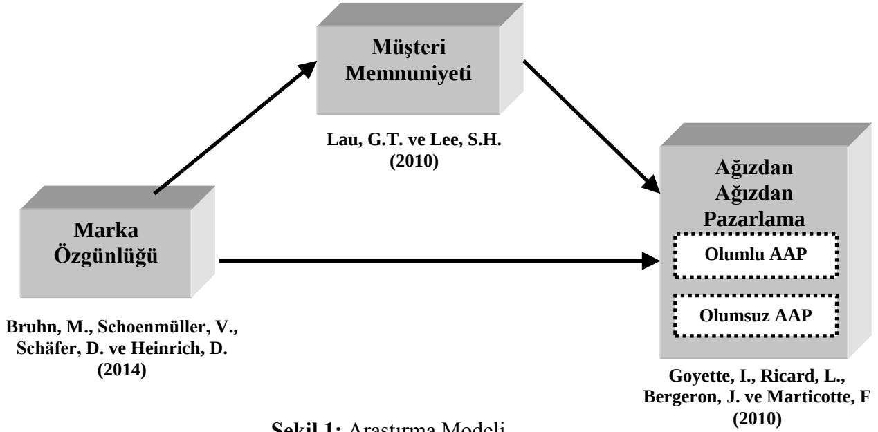
Şekil 1: Araştırma Modeli
