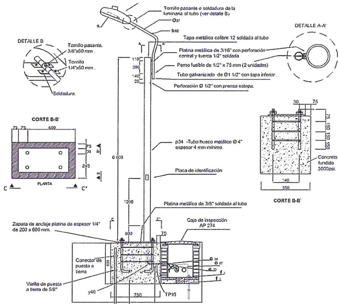
DETALLE DE LUMINARIAS
