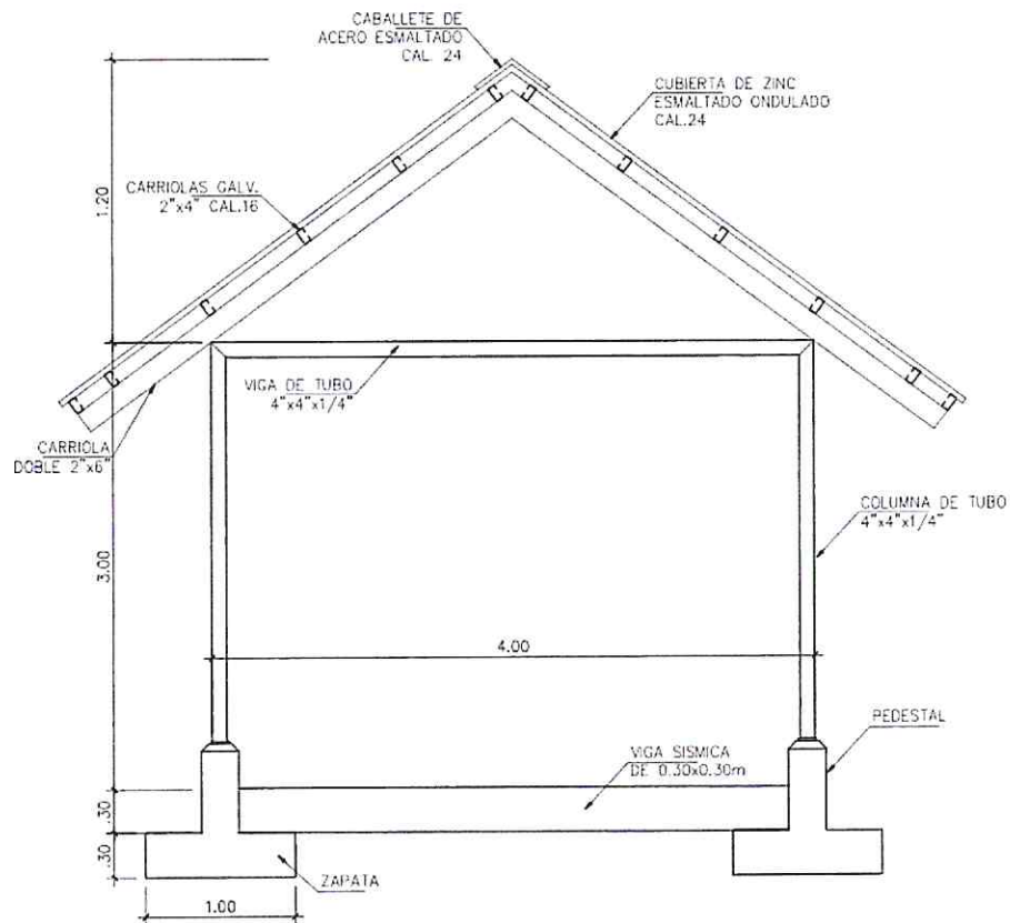
SECCIÓN GAZEBO
