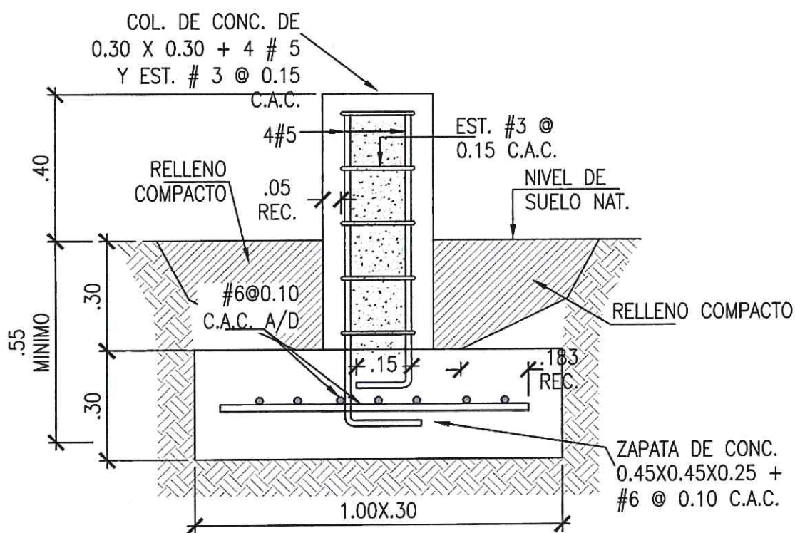
DETALLE DE PEDESTAL
