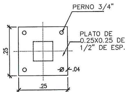
DETALLE ANCLAJE DE TUBO
