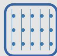
Precision
