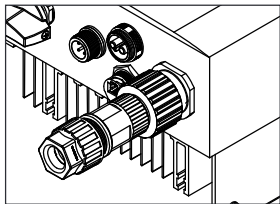
▲ Figura 4.18 Ligue o conector CA ao Inversor
