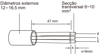
▲ Figura 4.15 Fios CA descarnados
