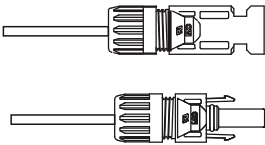
▲ Figura 4.11 Conector com porca aparafusada
