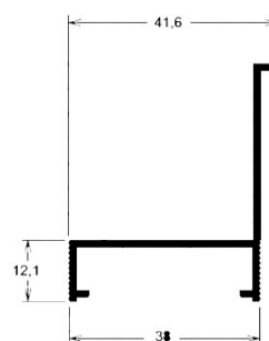
CM-098 0,382 kg/m
