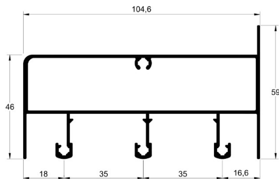
SU-019 1,770 kg/m
