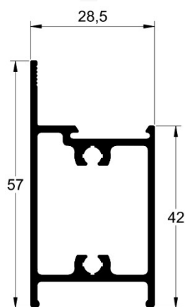
LG-058 0,831 kg/m
