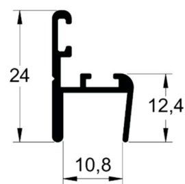
AL-17 0,309 kg/m
