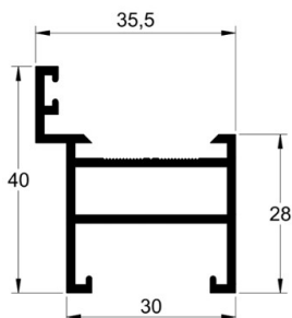
30-023 0,588 kg/m
