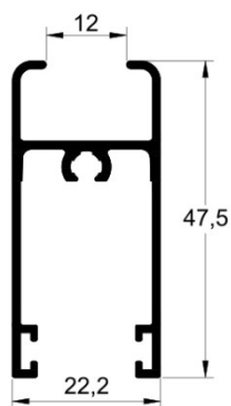
SU-186 0,498 kg/m
