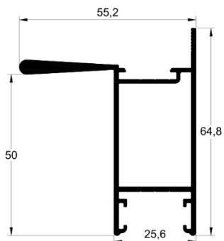
SU-280 0,928 kg/m
