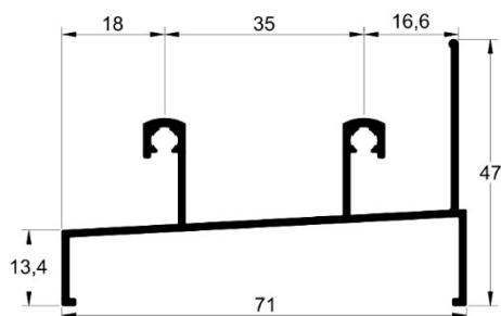
SU-002 0,679 kg/m
