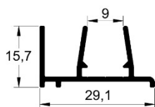
SU-008 0,257 kg/m
