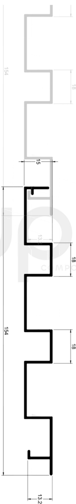
TLB-377 0,851 kg/m
