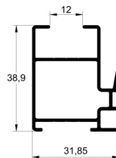
SU-056 0,464 kg/m
