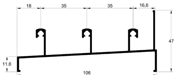
SU-011 0,888 kg/m
