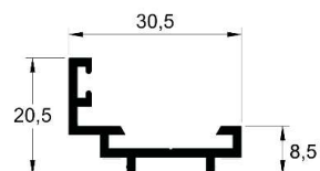
25-548 0,254 kg/m
