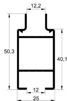
SU-190 0,536 kg/m
