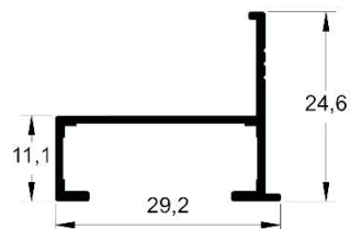
CM-110 0,183 kg/m
