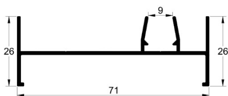
SU-003 0,571 kg/m
