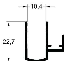
MH-69 0,266 kg/m
