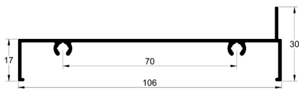
SU-018 0,669 kg/m
