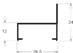
CM-200 0,179 kg/m
