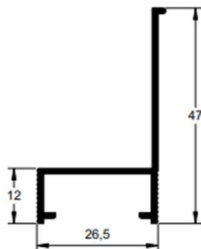
CM-151 0,309 kg/m
