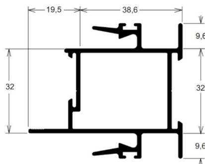
LG-162 1,206 kg/m
