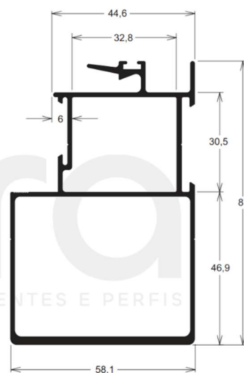
LG-052 1,619 kg/m
