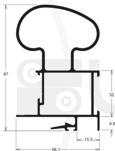
LG-021 1,716 kg/m
