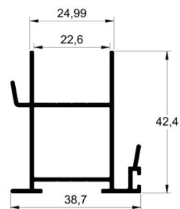
SU-069 0,496 kg/m
