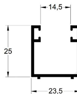
BX-054 0,278 kg/m
