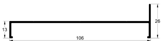
SU-012 0,497 kg/m
