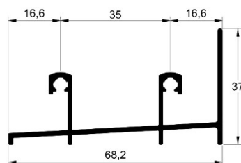
SU-228 0,678 kg/m
