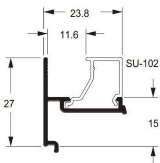
SU-292 0,220 kg/m
