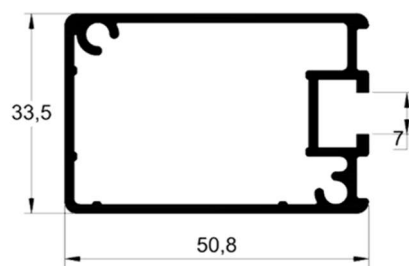
CG-077 0,733 kg/m
