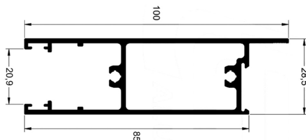
LG-007 1,121 kg/m
