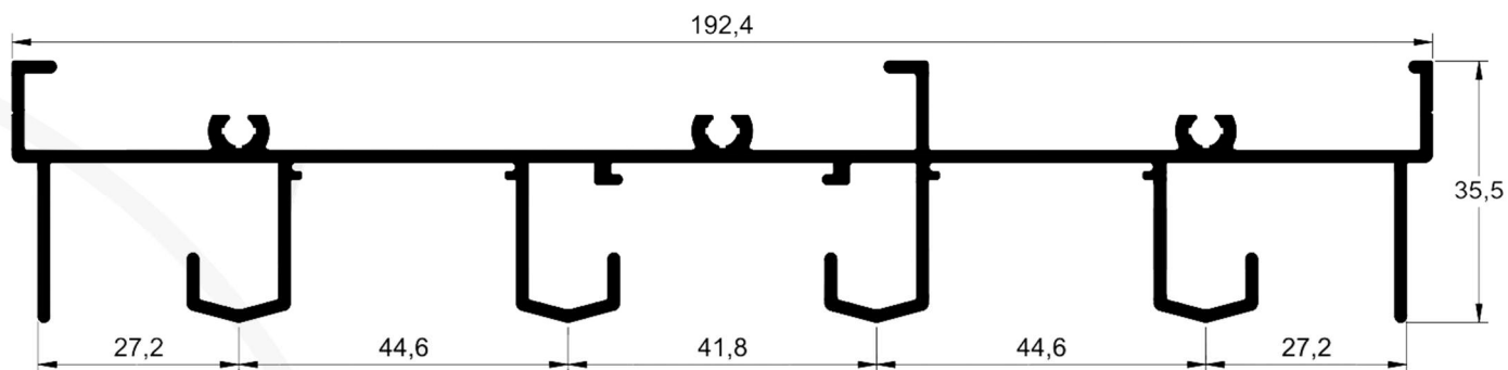
LG-070 2,101 kg/m
