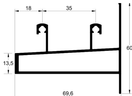
SU-006 1,086 kg/m
