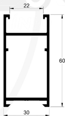
30-077 0,828 kg/m
