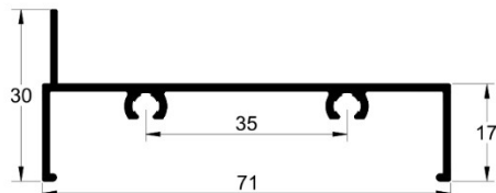
SU-004 0,489 kg/m
