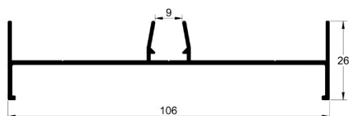
SU-014 0,673 kg/m
