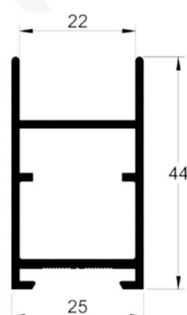
A-207 0,542 kg/m
