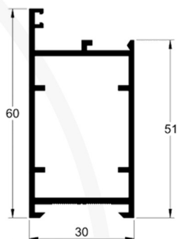
30-026 0,787 kg/m
