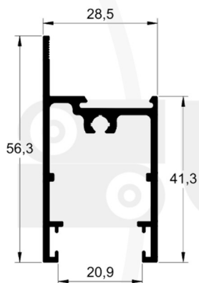
LG-006 0,686 kg/m
