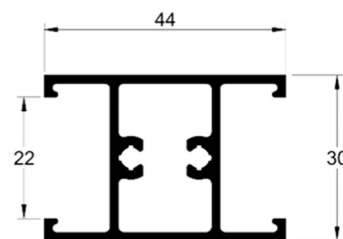
30-079 0,744 kg/m
