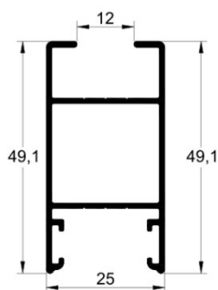
SU-055 0,545 kg/m
