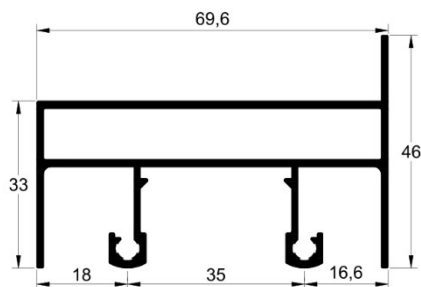
SU-005 1,080 kg/m
