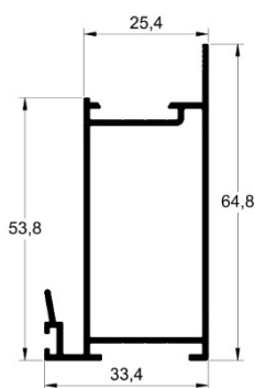
SU-242 0,636 kg/m
