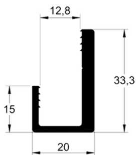
CG-075 0,533 kg/m
