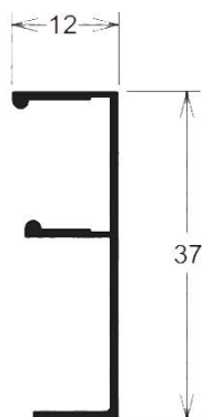
MP-347 0,188 kg/m
