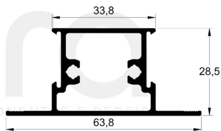
LG-055 0,757 kg/m
