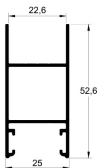
SU-068 0,498 kg/m
