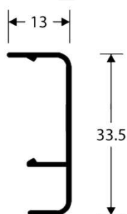
CM-130 0,166 kg/m
