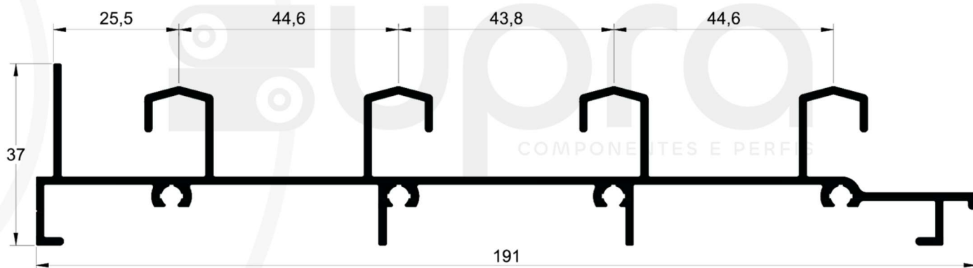
LG-071 2,062 kg/m
