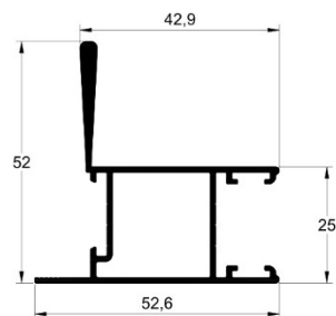
SU-250 0,713 kg/m
