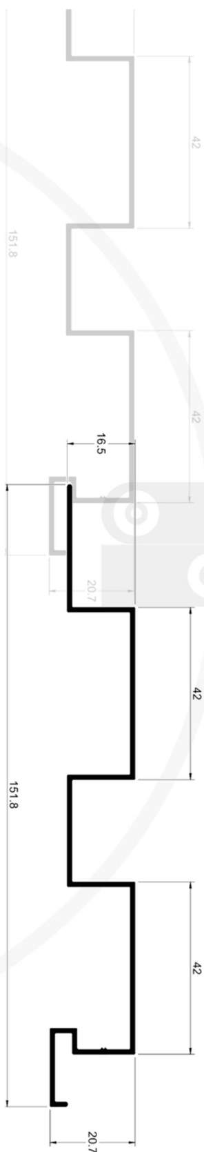
TLB-376 0,719 kg/m
