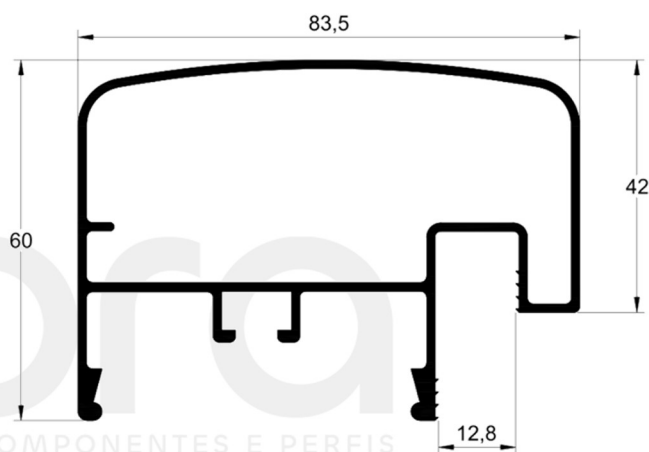
CG-083 1,466 kg/m
