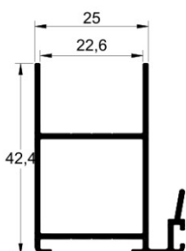
SU-070 0,525 kg/m
