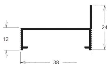
CM-060 0,254 kg/m
