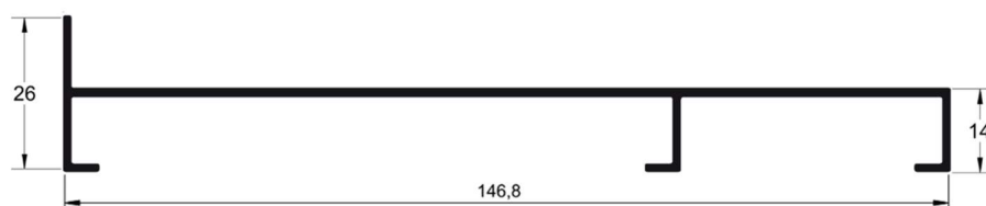
LG-158 0,884 kg/m
