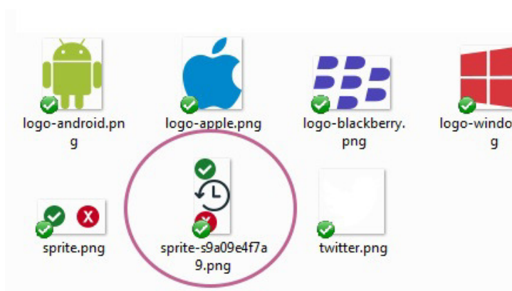
Figura 9.13: Sprite teste
