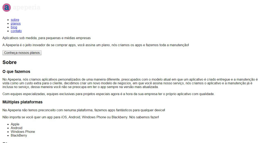
Figura 5.3: Layout sumiu
