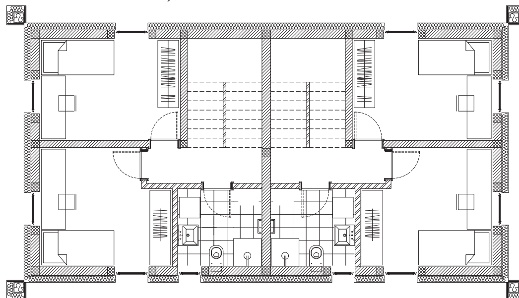
TLORIS NADSTROPJA
