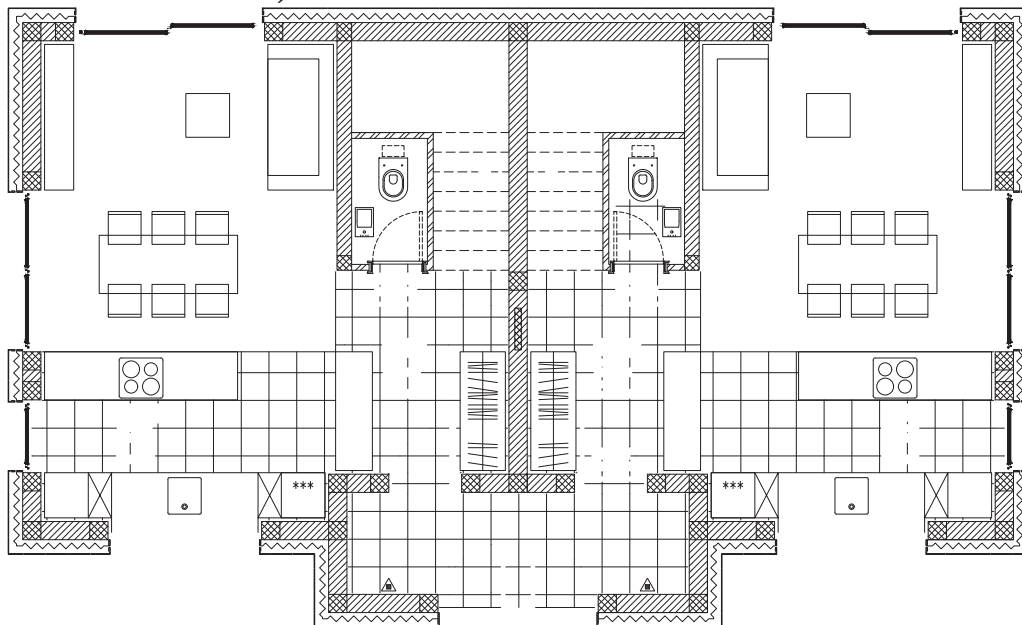
TLORIS PRITLIČJA
