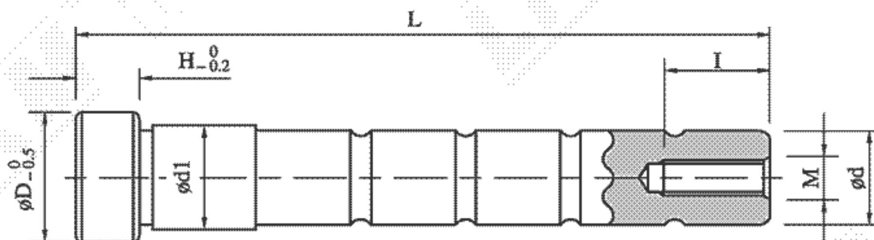
尺寸公差 Dimension
