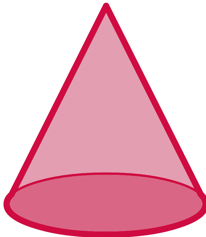
Cone
