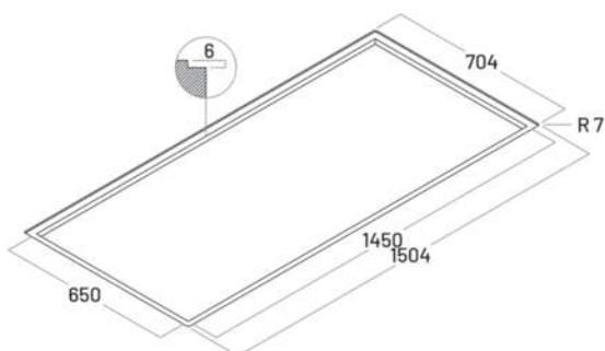
Foro d'incasso per montaggio filotop Cut out flush mounting
