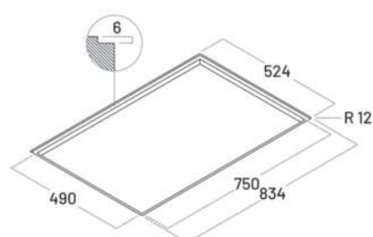
Foro d'incasso per montaggio filotop Cut out flush mounting
