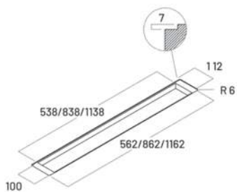
Foro d'incasso Cut out
