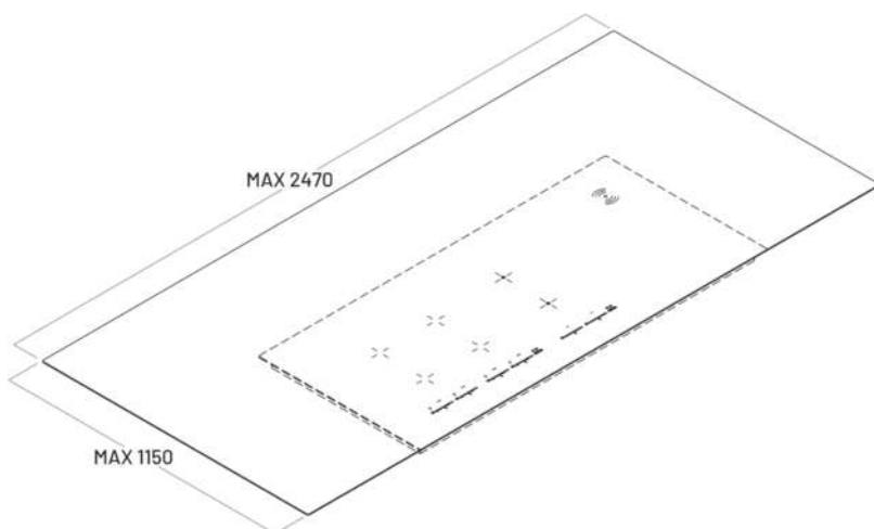
Versione con dimensioni personalizzate Customized size version
