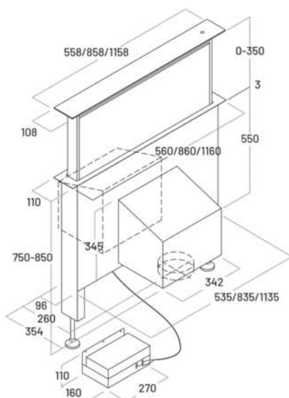
Foro d'incasso Cut out
