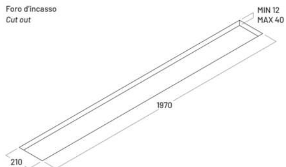
VERSIONE STANDARD STANDARD VERSION
