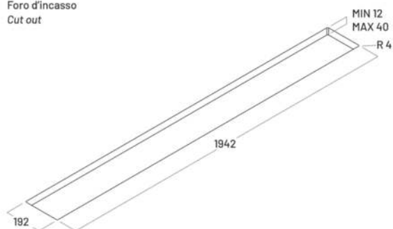
VERSIONE PANNELLABILE VERSION TO BE PANELED
