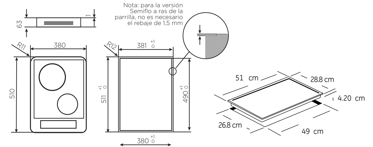
PVP3021 - 30 CM
