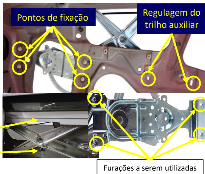
Trilho principal do vidro
