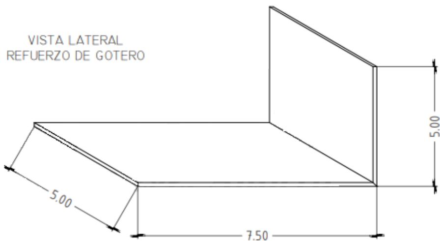
ISOMÉTRICO REFUERZO DE GOTERO
