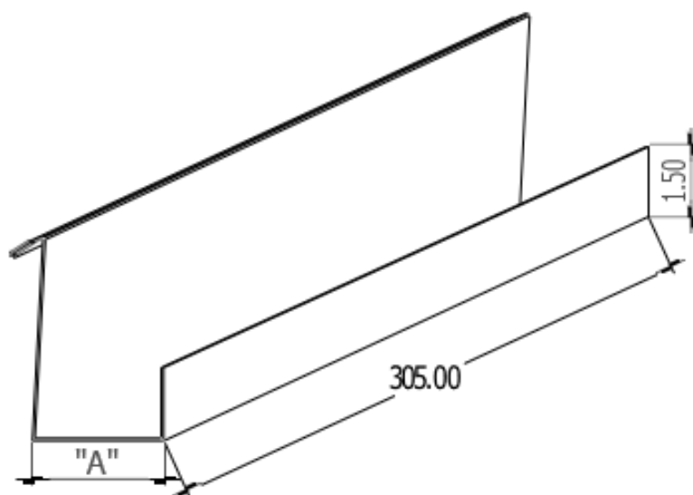
ISOMÉTRICO CANAL TAPÓN PARA INSULFOIL
