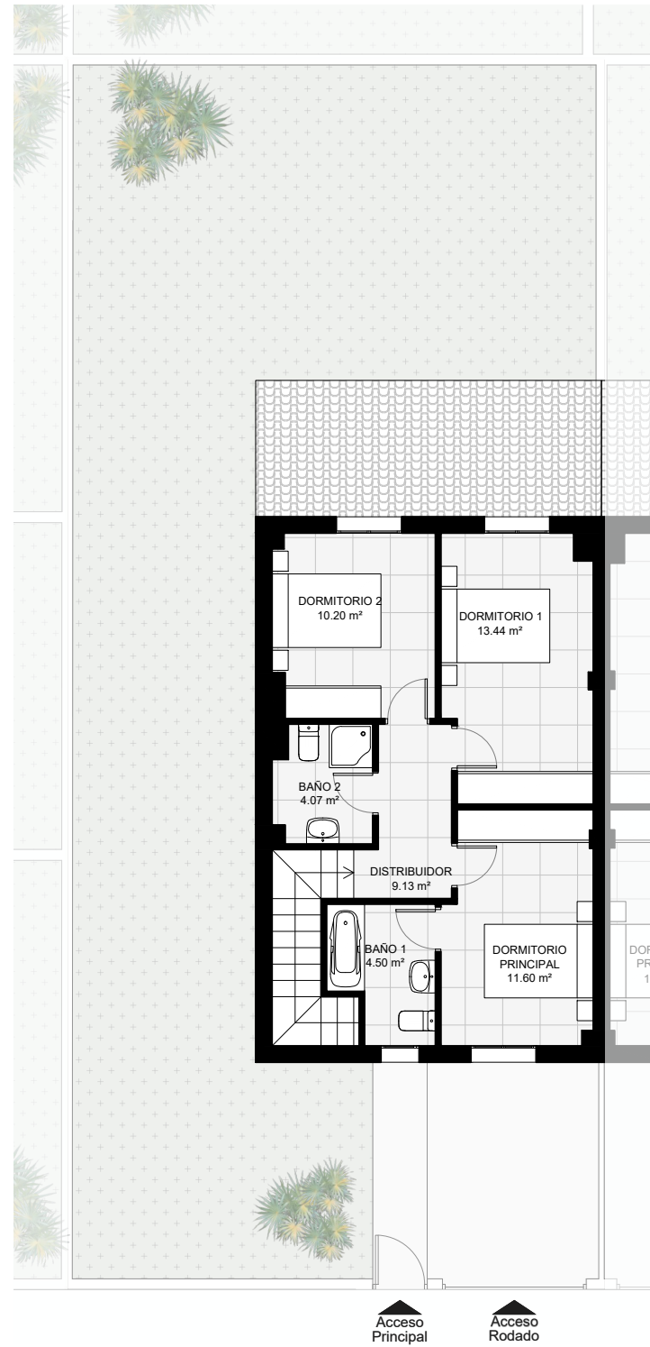
PLANTA PRIMERA
