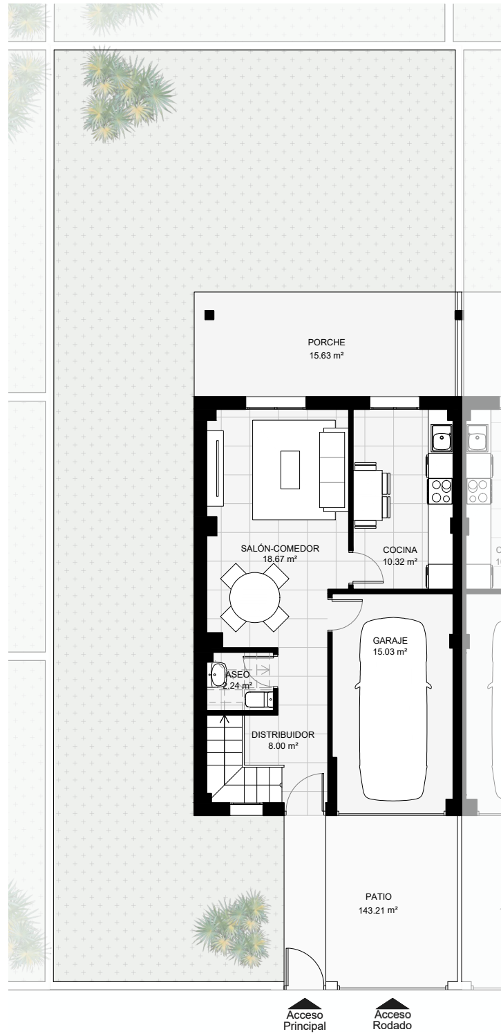
PLANTA BAJA
