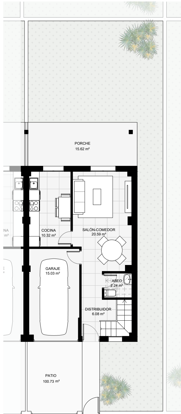
PLANTA BAJA
