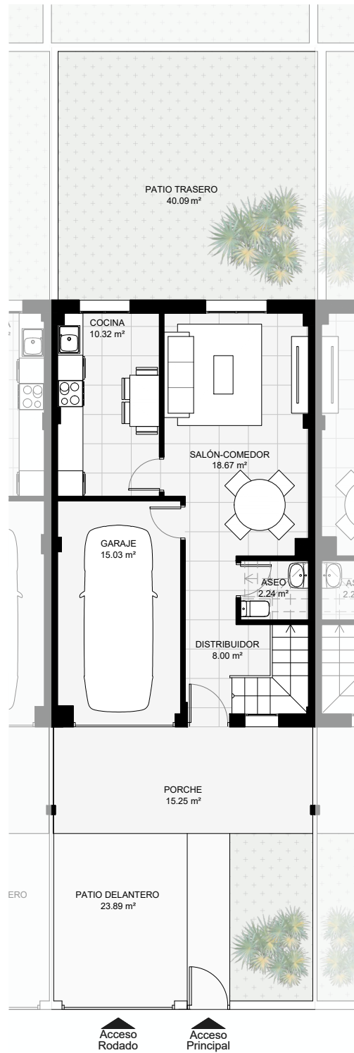
PLANTA BAJA
