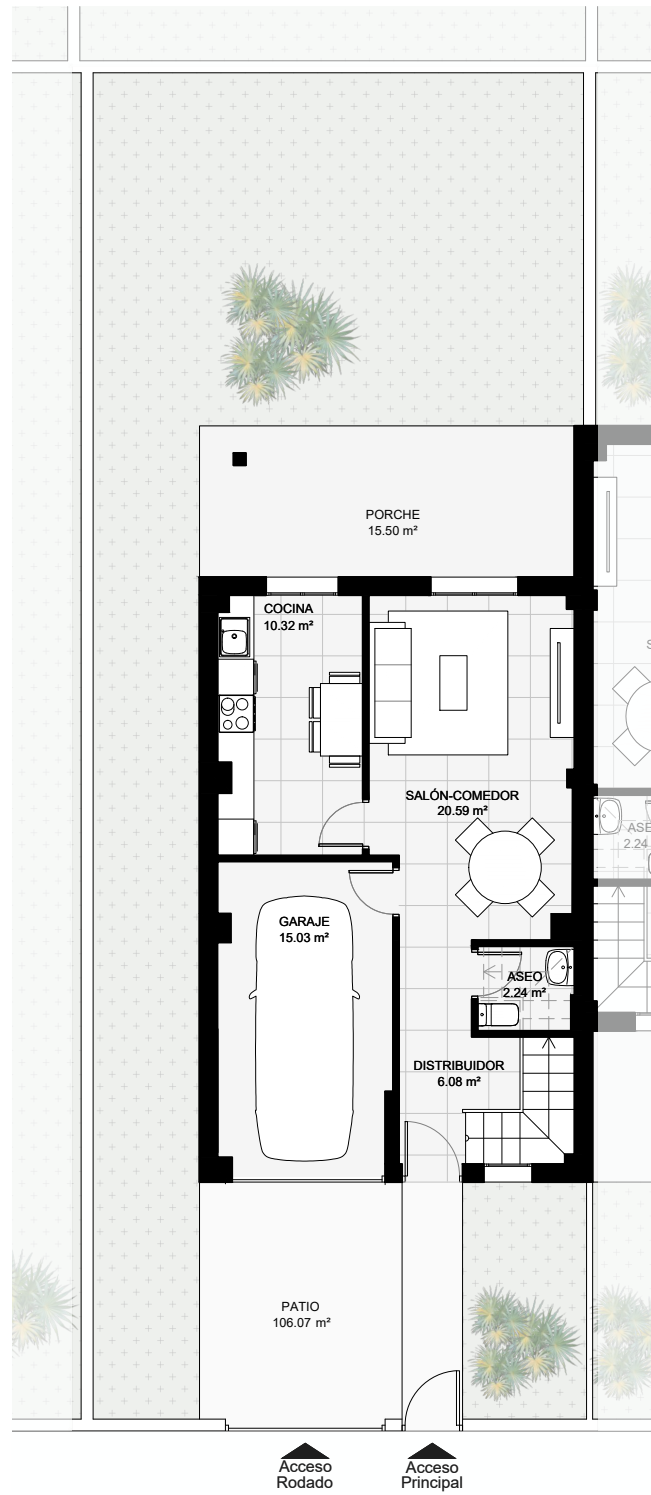
PLANTA BAJA
