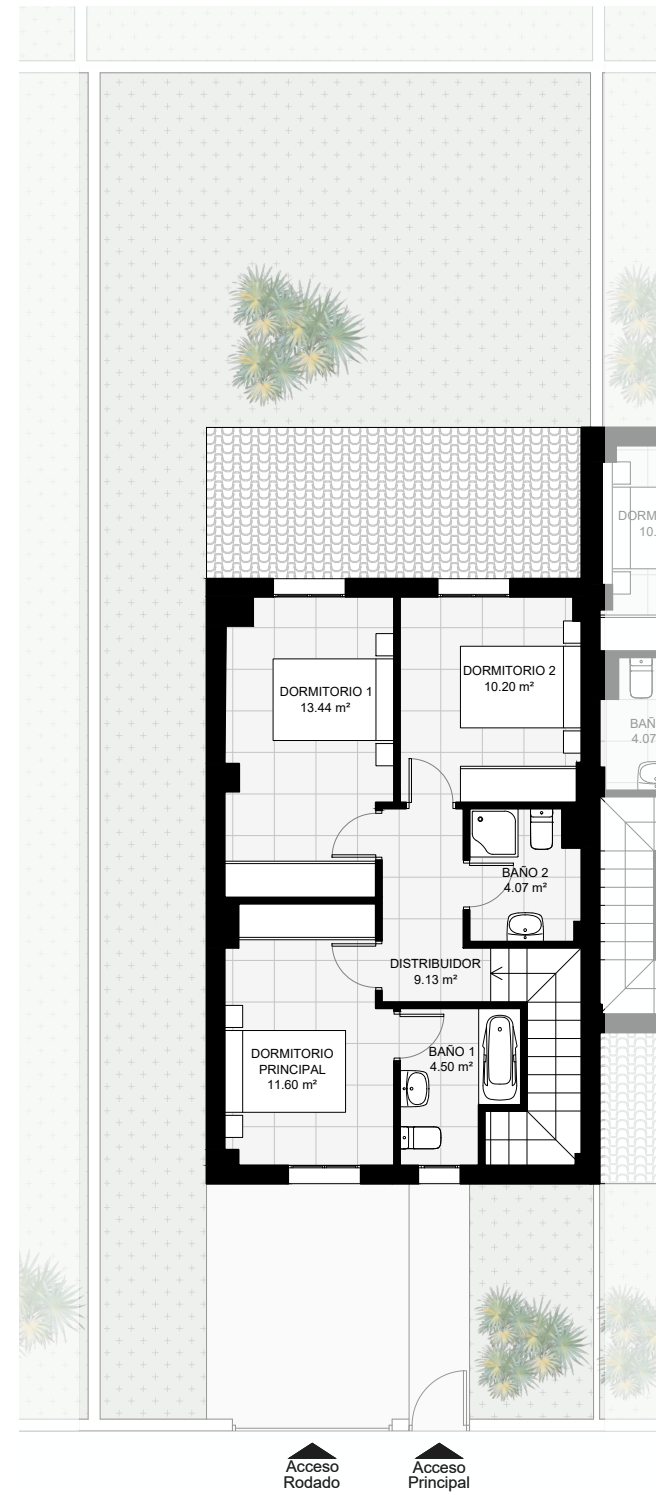
PLANTA PRIMERA
