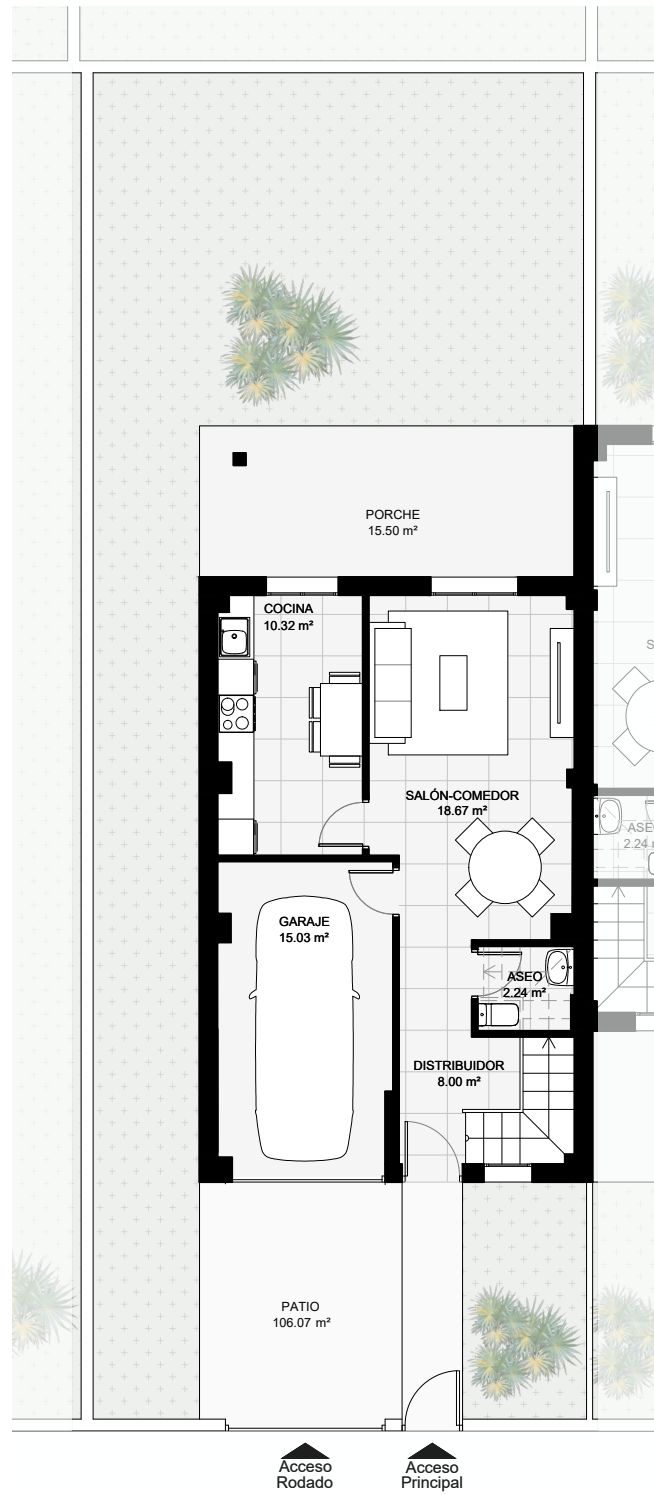
PLANTA BAJA
