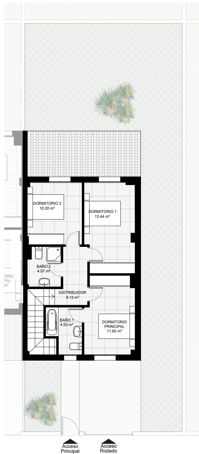
PLANTA PRIMERA
