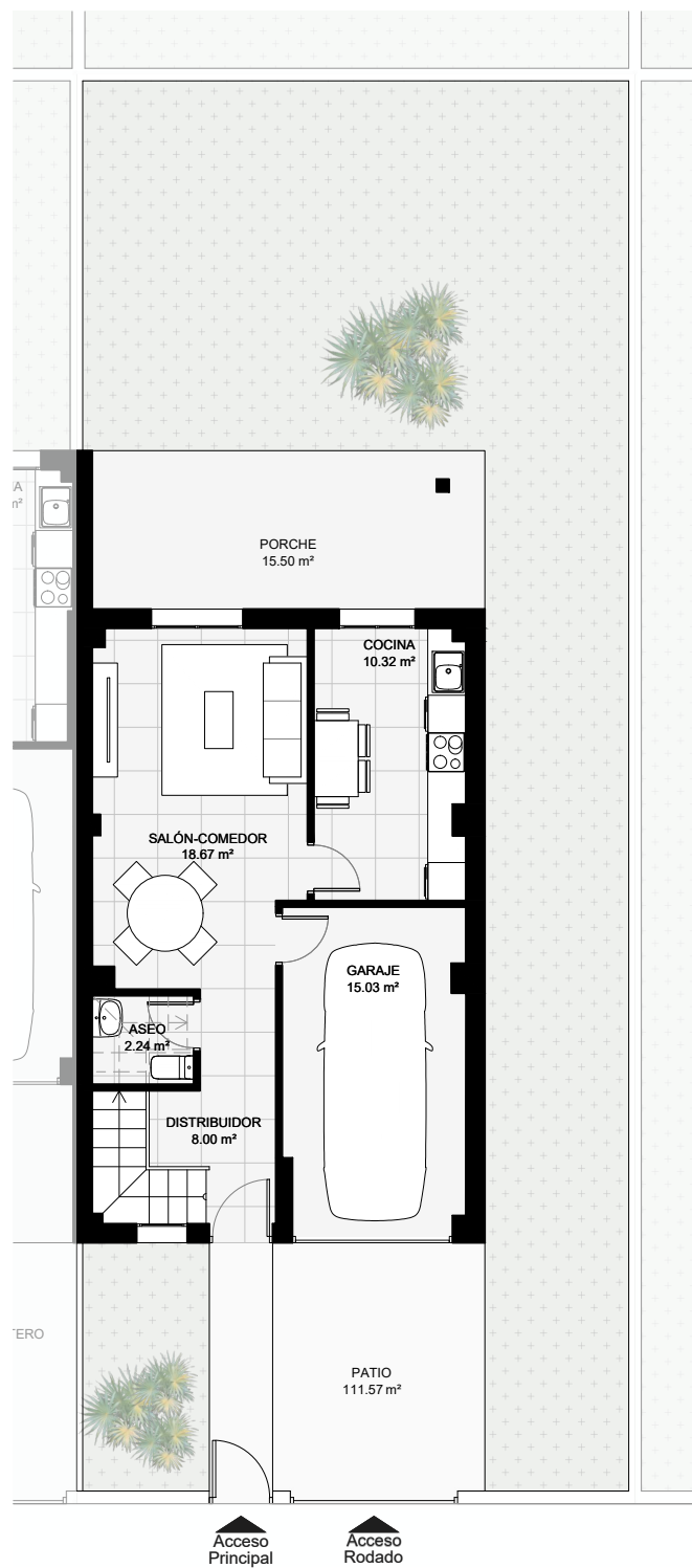
PLANTA BAJA
