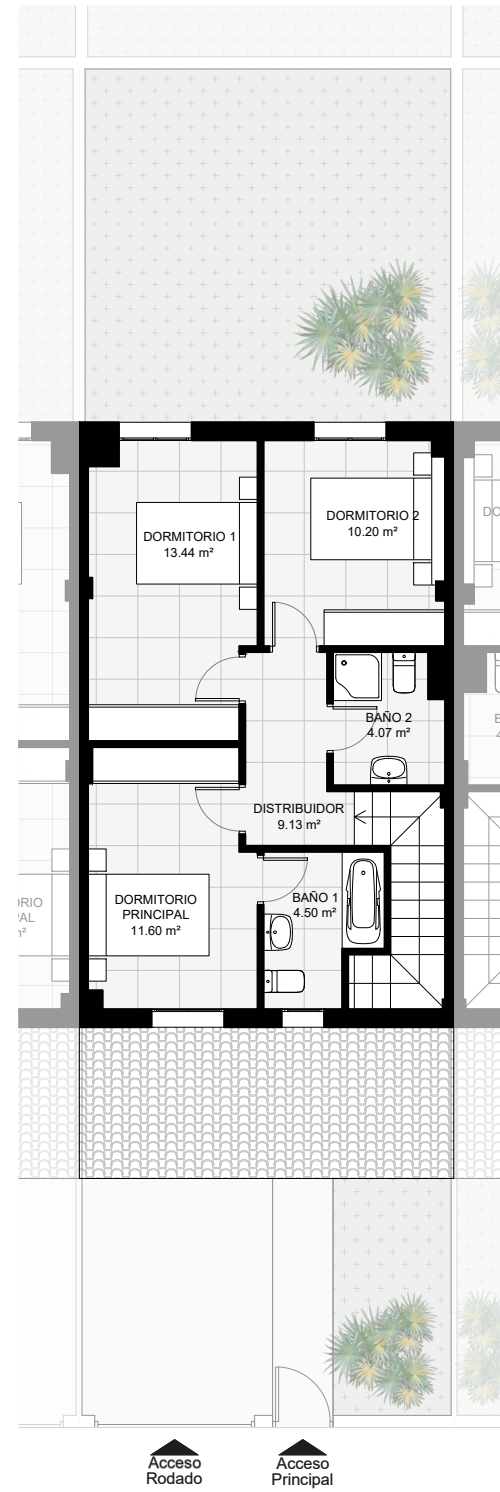
PLANTA PRIMERA
