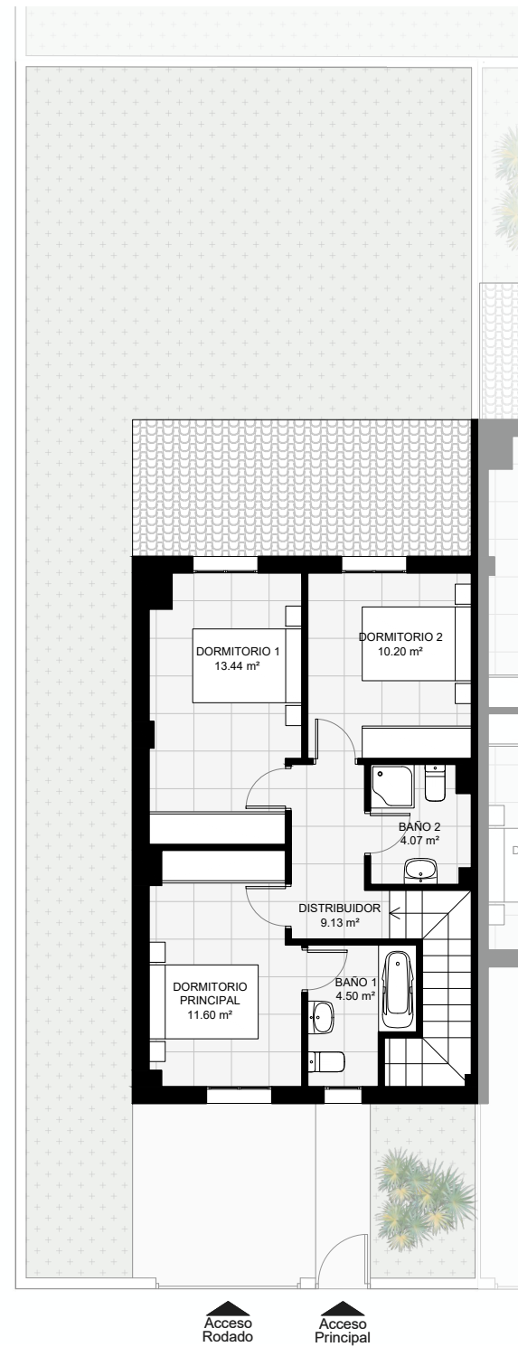
PLANTA PRIMERA
