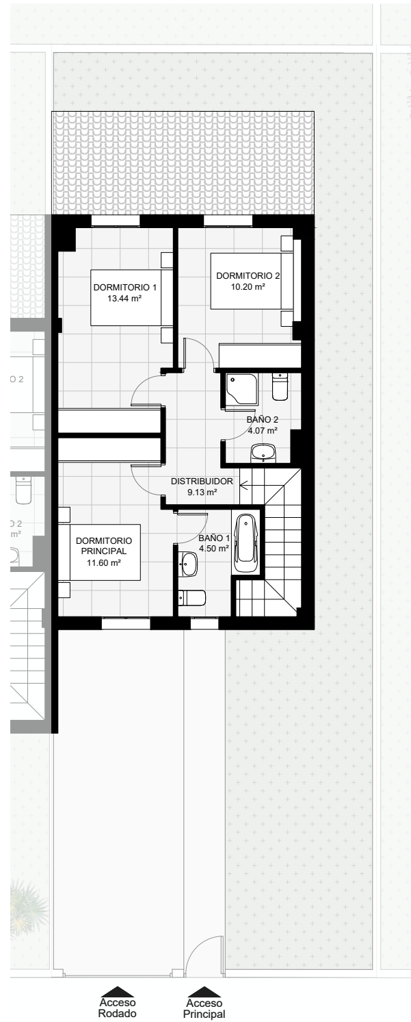
PLANTA PRIMERA
