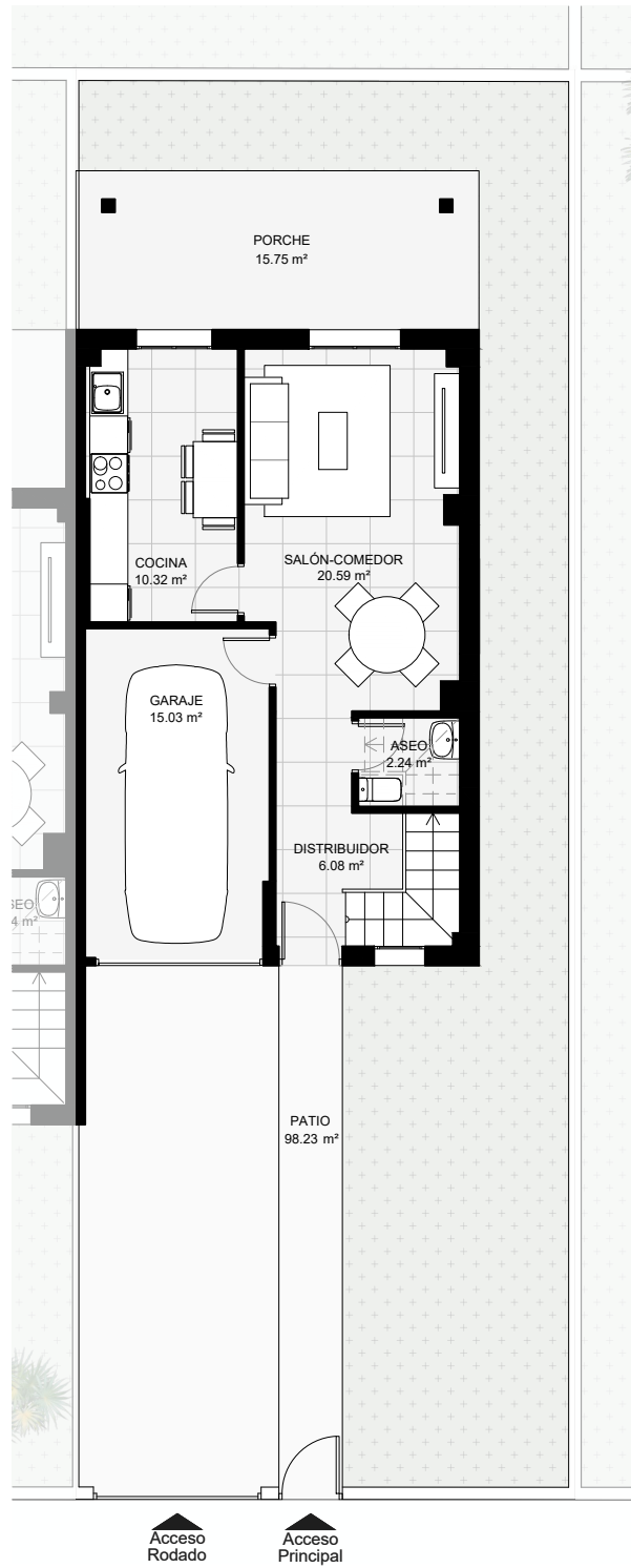
PLANTA BAJA
