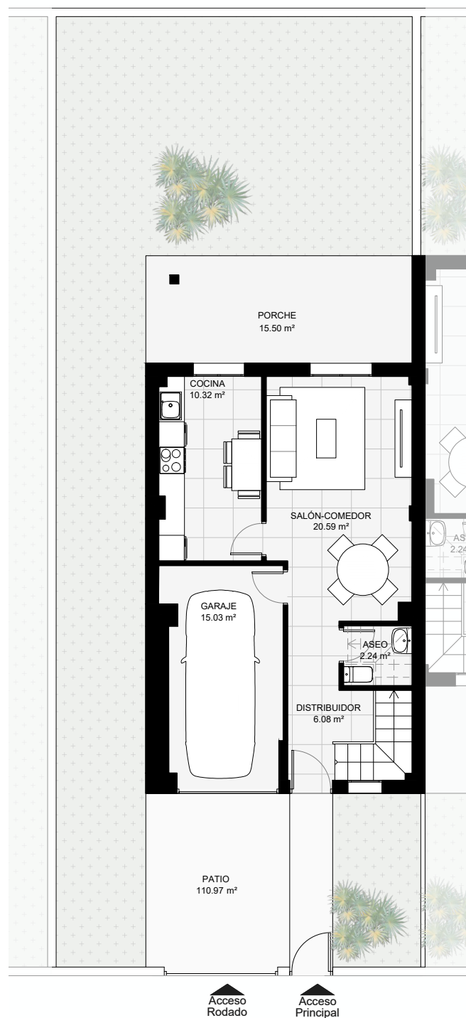
PLANTA BAJA
