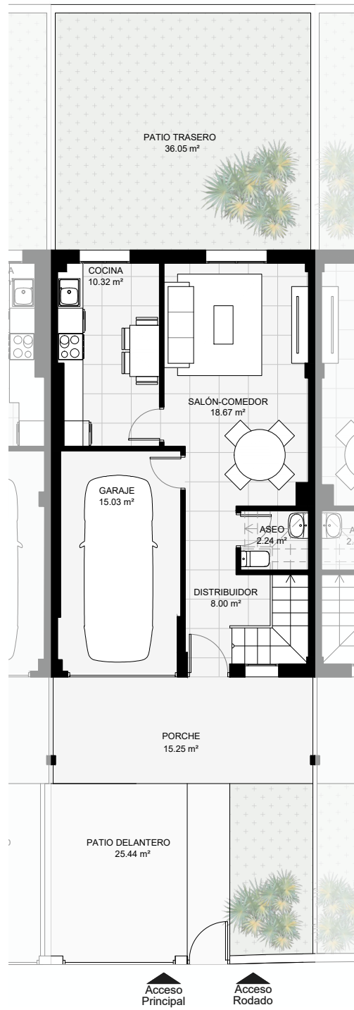
PLANTA BAJA
