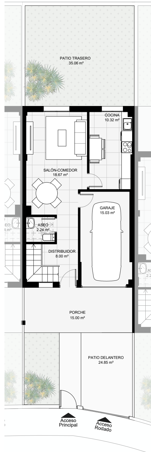
PLANTA BAJA
