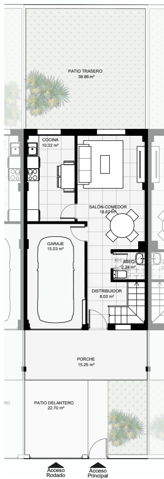
PLANTA BAJA
