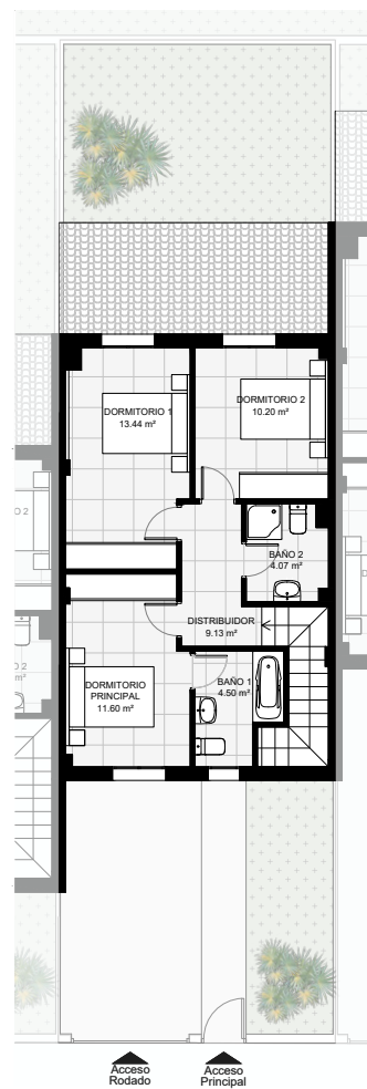
PLANTA PRIMERA
