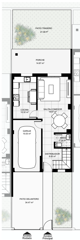
PLANTA BAJA
