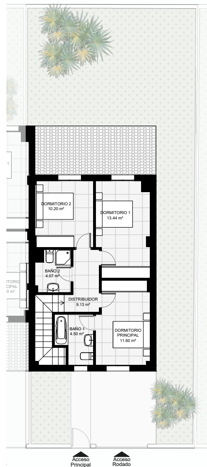
PLANTA PRIMERA
