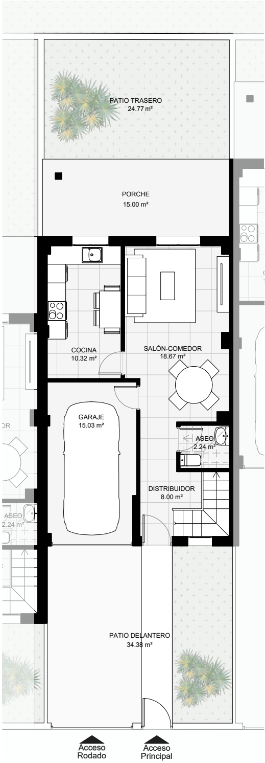
PLANTA BAJA
