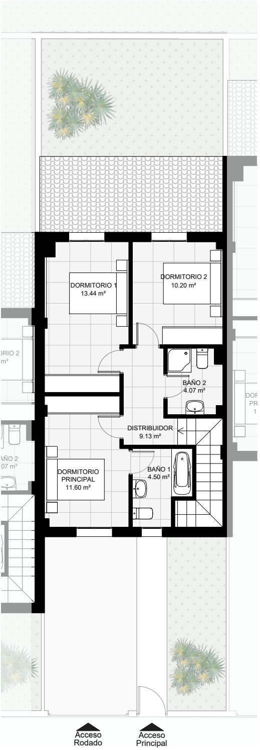
PLANTA PRIMERA
