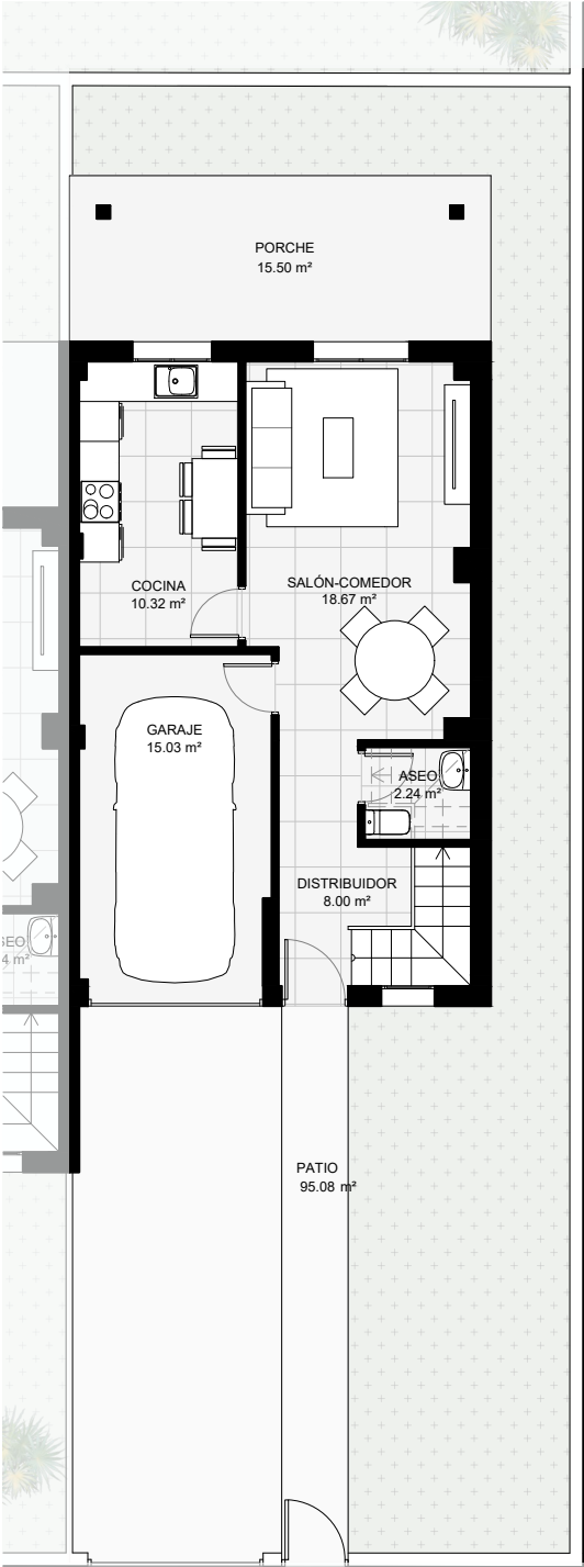
PLANTA BAJA
