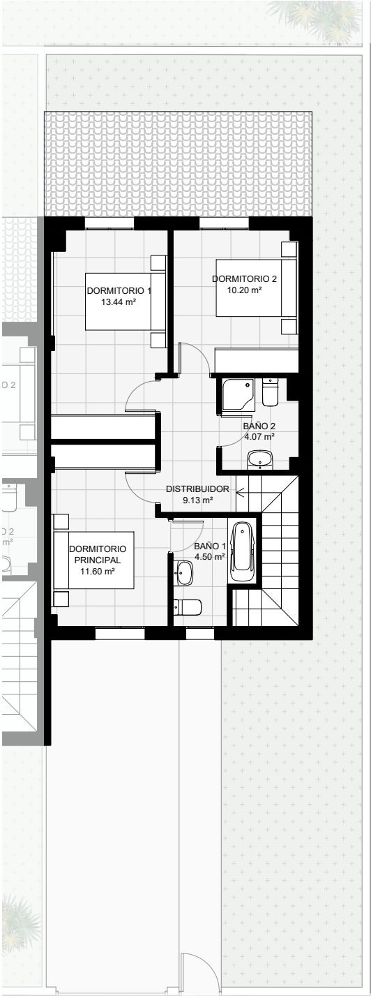
PLANTA PRIMERA
