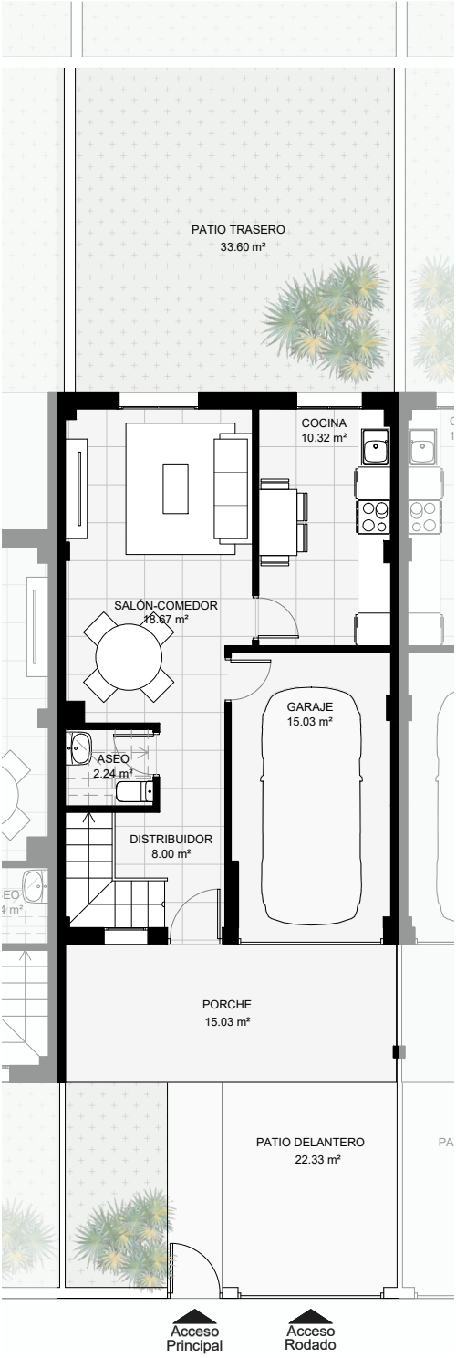
PLANTA BAJA
