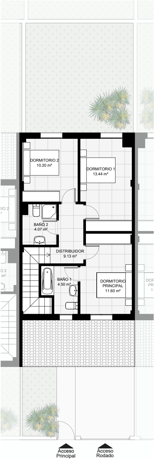
PLANTA PRIMERA
