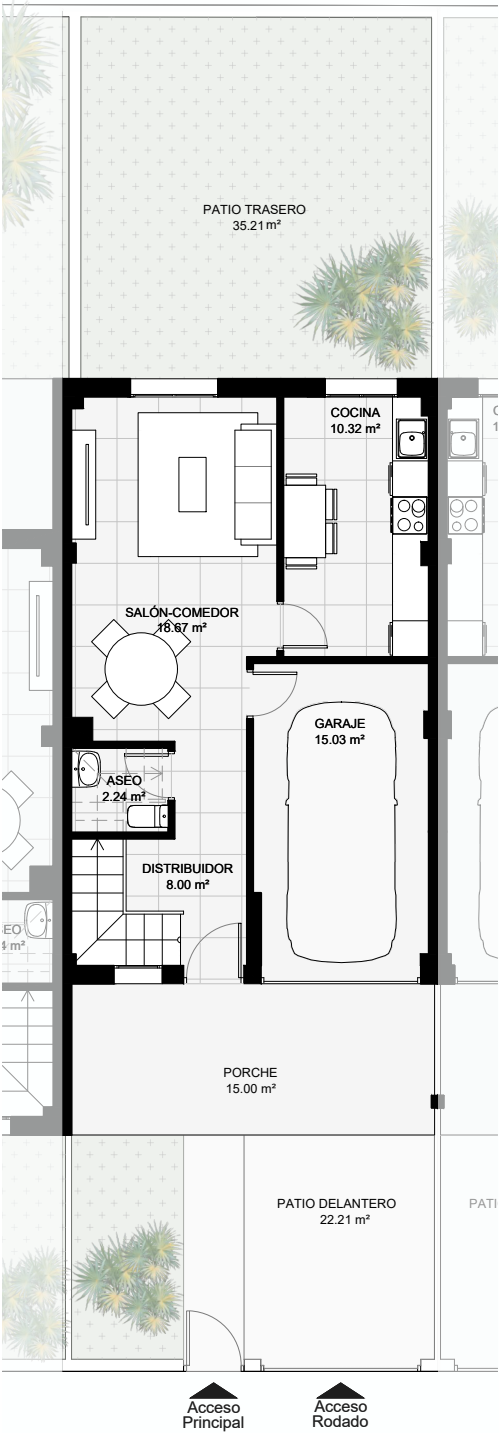
PLANTA BAJA
