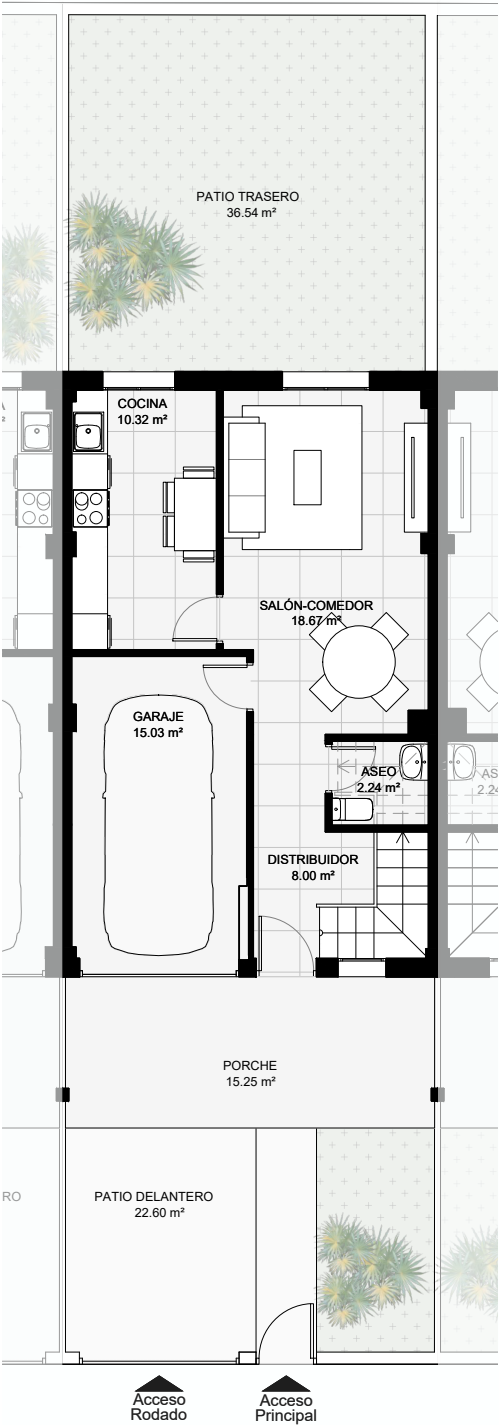
PLANTA BAJA
