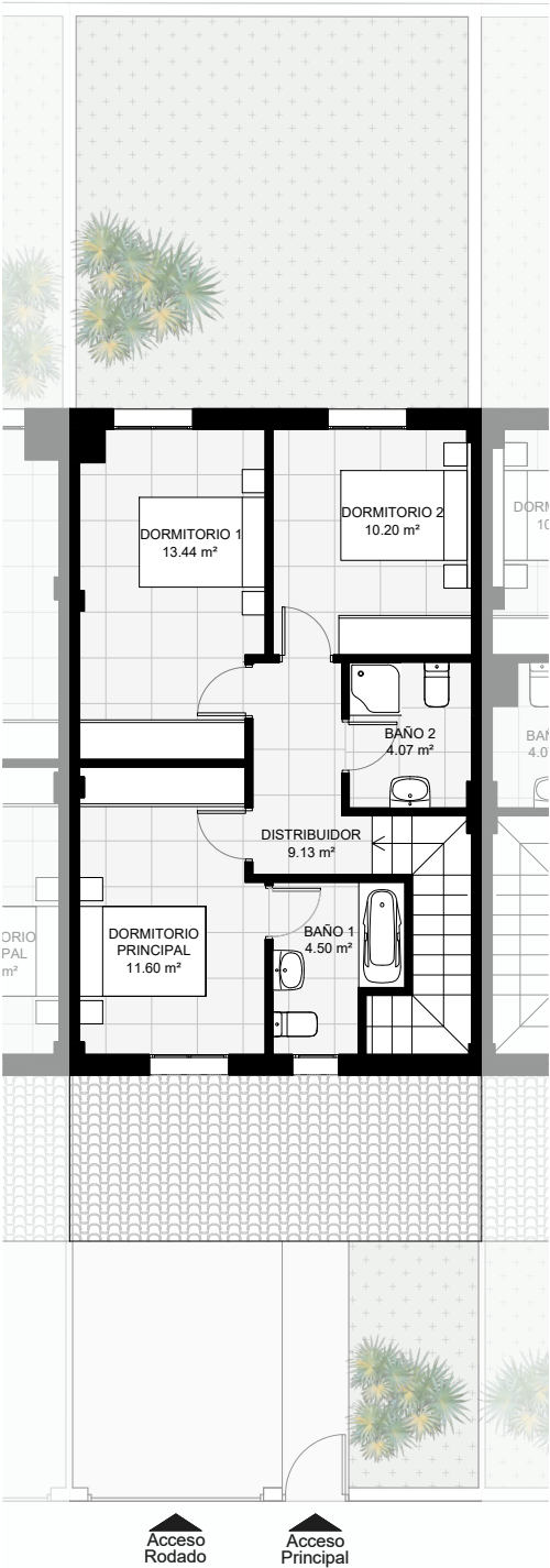
PLANTA PRIMERA
