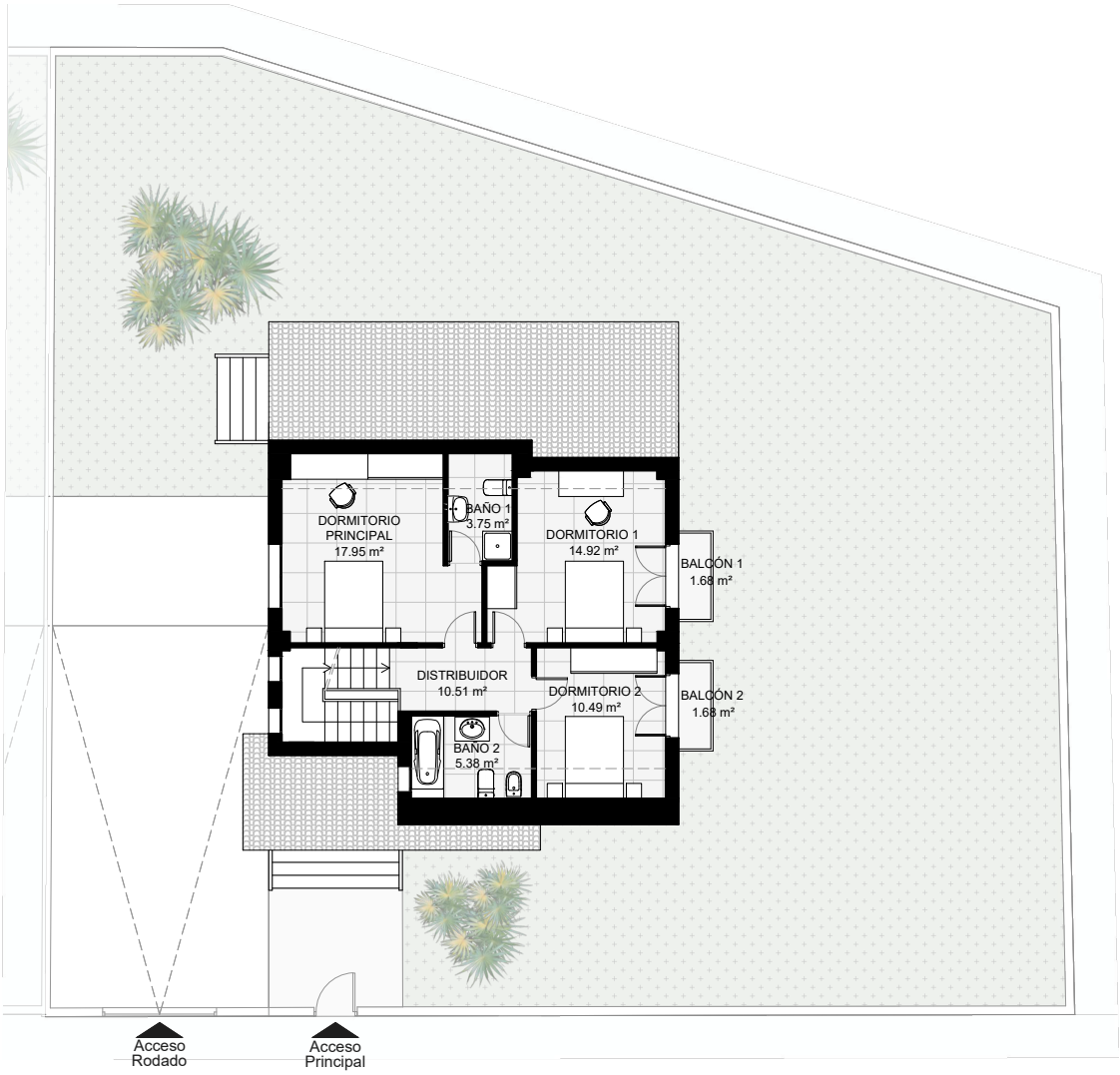
PLANTA PRIMERA
