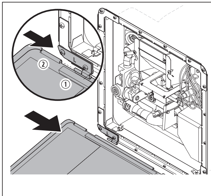
14 Glissement de la trappe d'accès sur la charnière gauche
