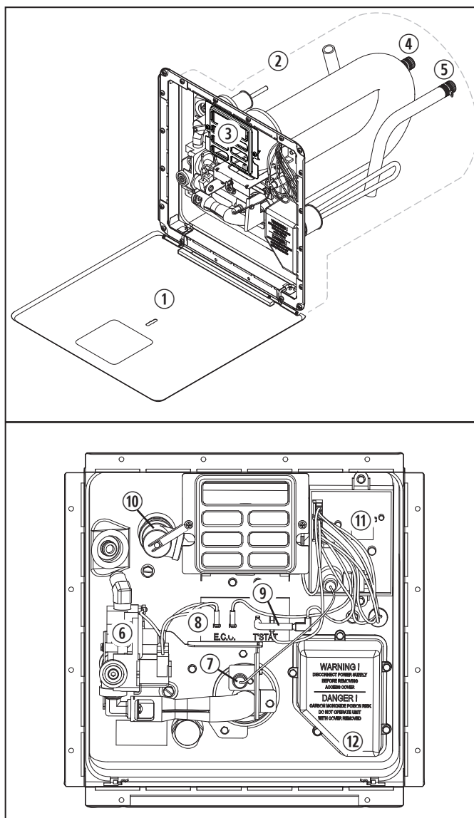
1 Emplacements des composants
