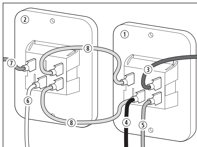
10 Câblage d'un interrupteur simple à fonction combinée
