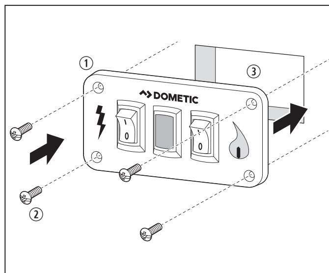
8 Installation de l'interrupteur double
