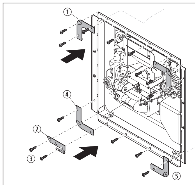
13 Fixer les équerres de fixation et la bride
