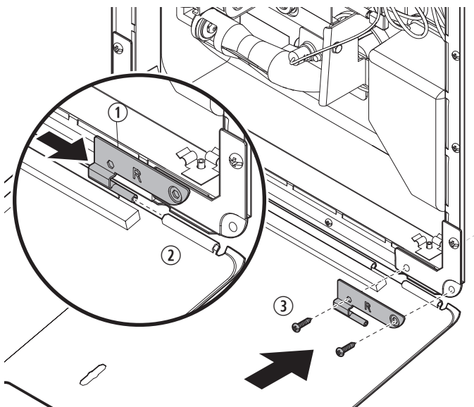
15 Fixation de la charnière droite
