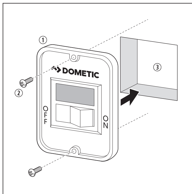
7 Installation de l'interrupteur simple
