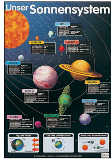
Unser Sonnensystem
