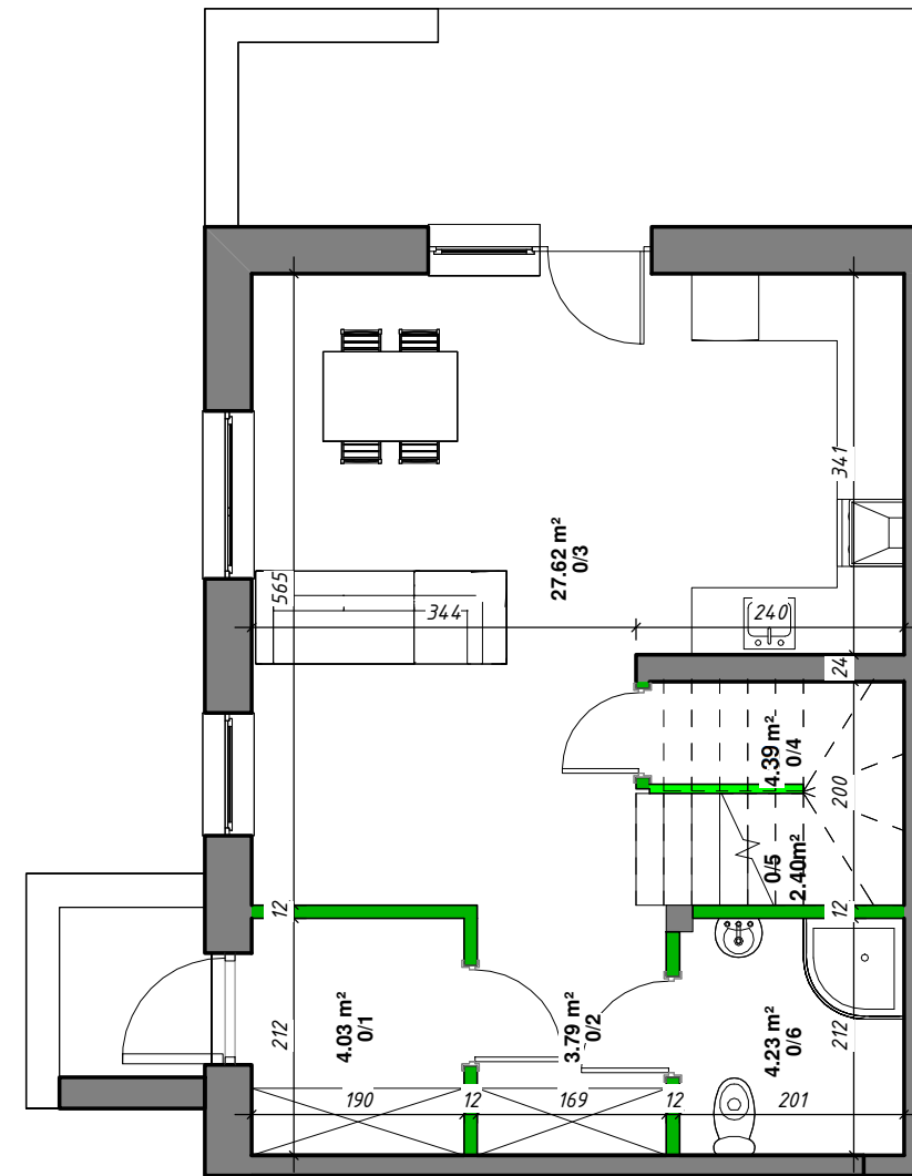
Rzut parteru
