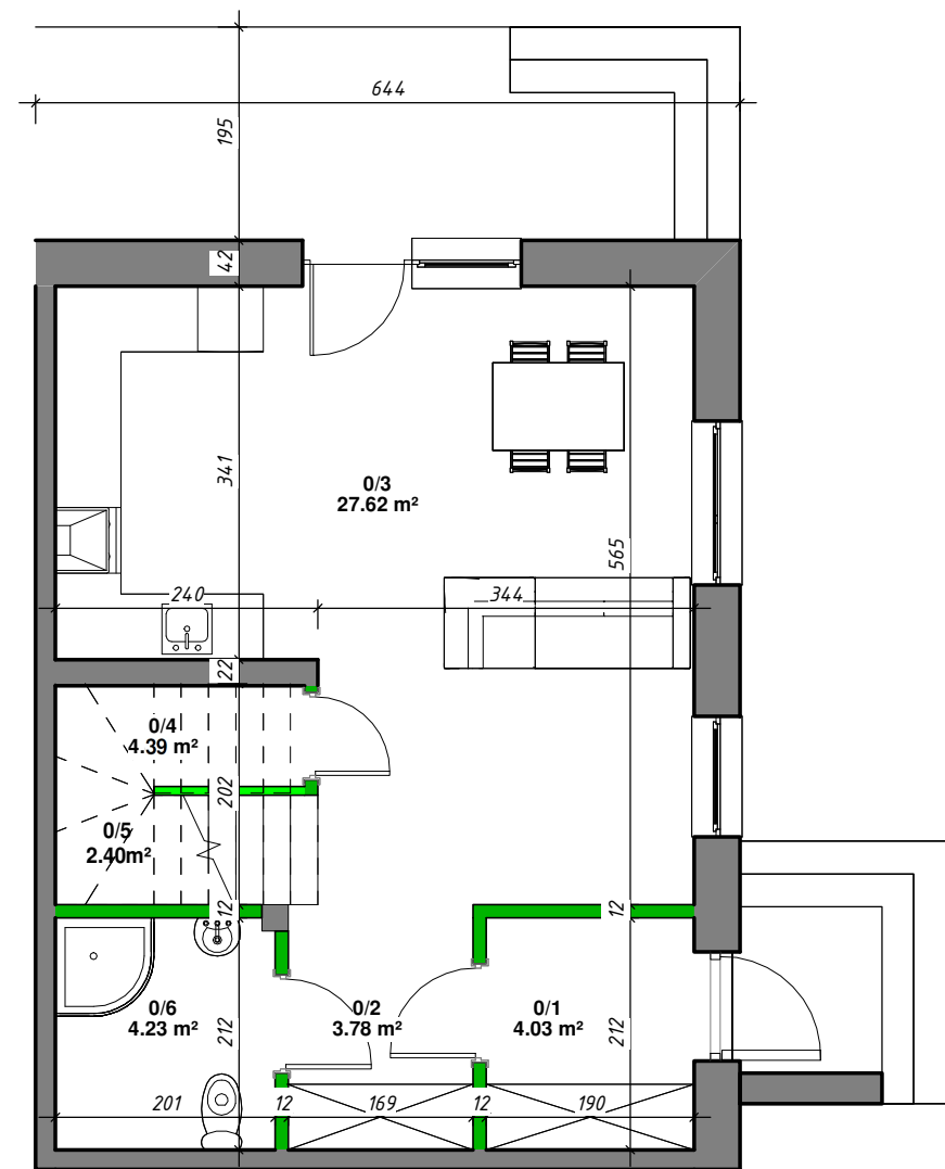
Rzut parteru
