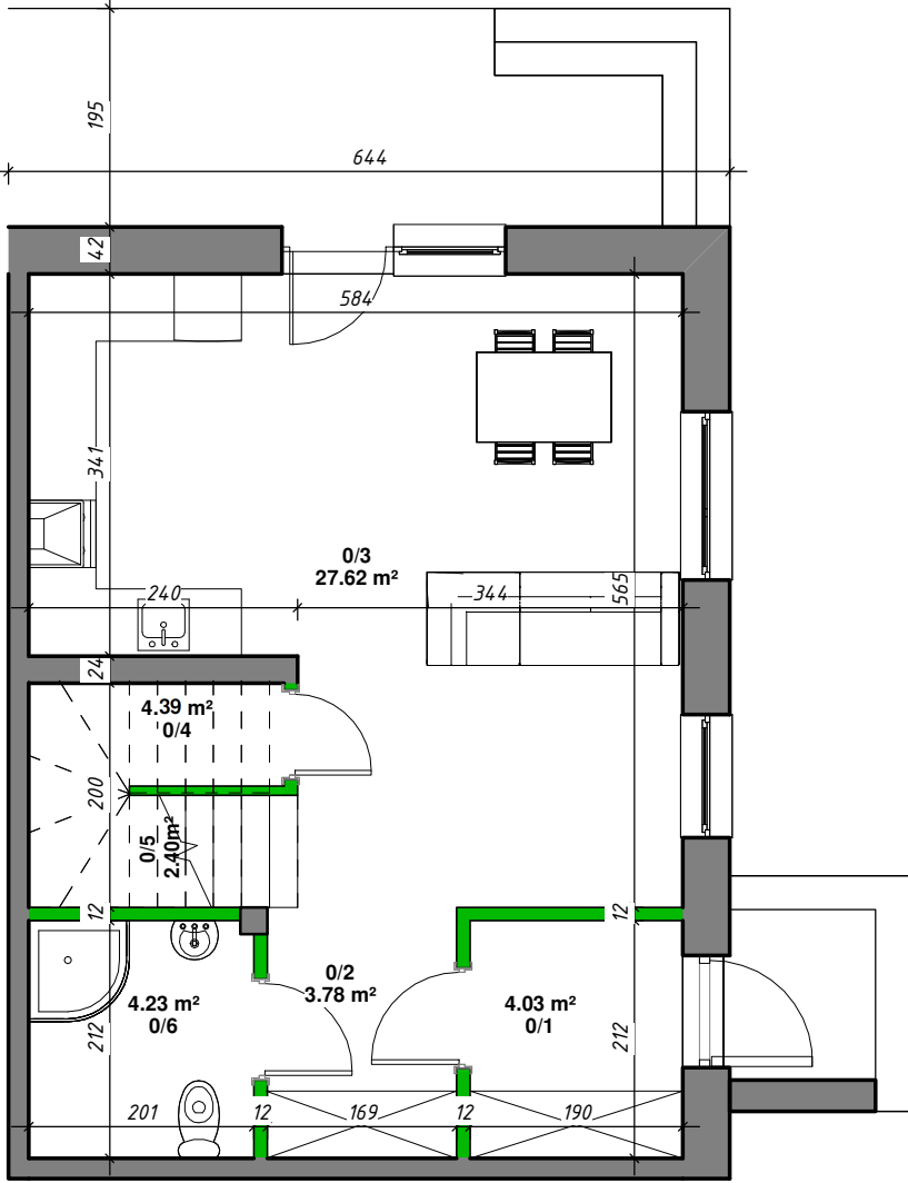
Rzut parteru
