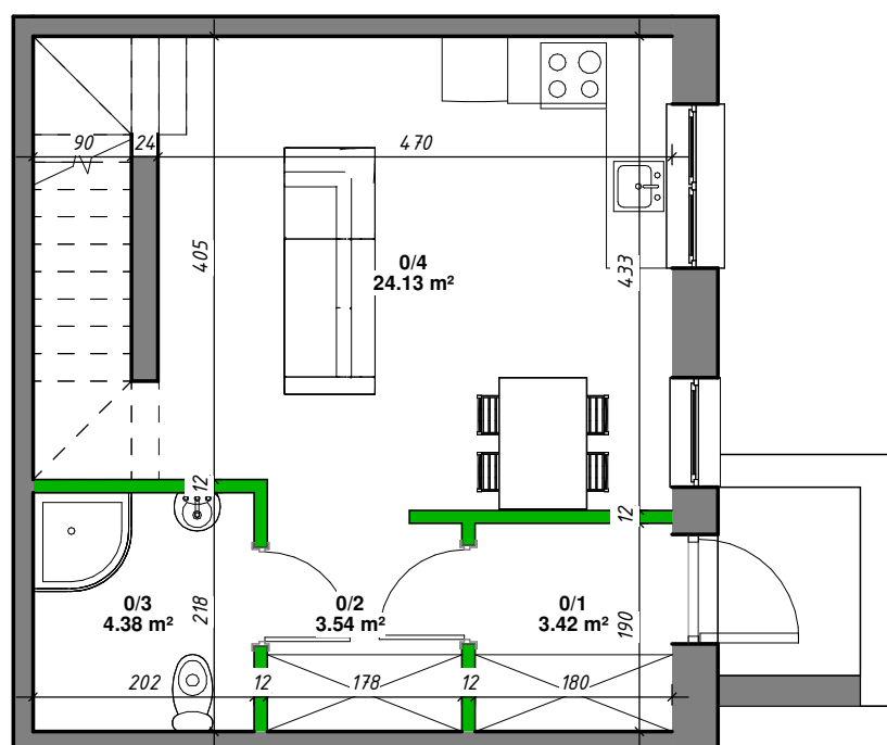
Rzut parteru
