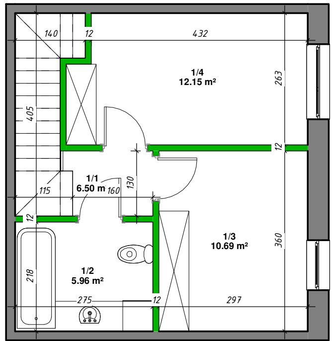
Rzut piętra
