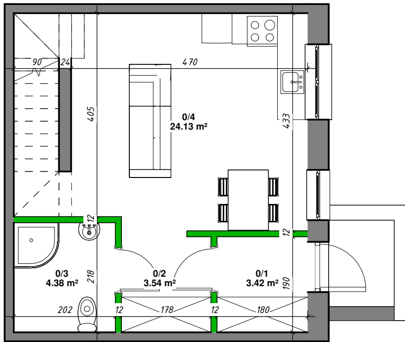
Rzut parteru
