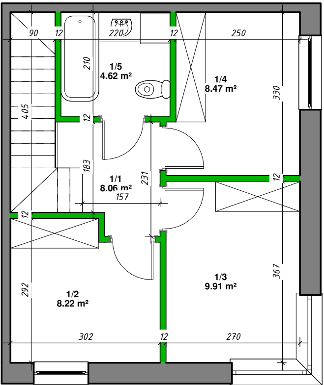
Rzut piętra
