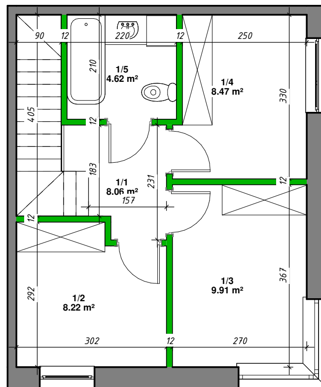
Rzut piętra
