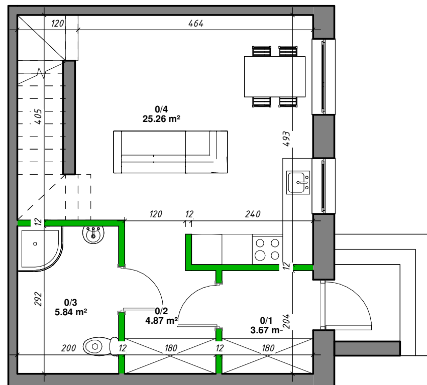
Rzut parteru
