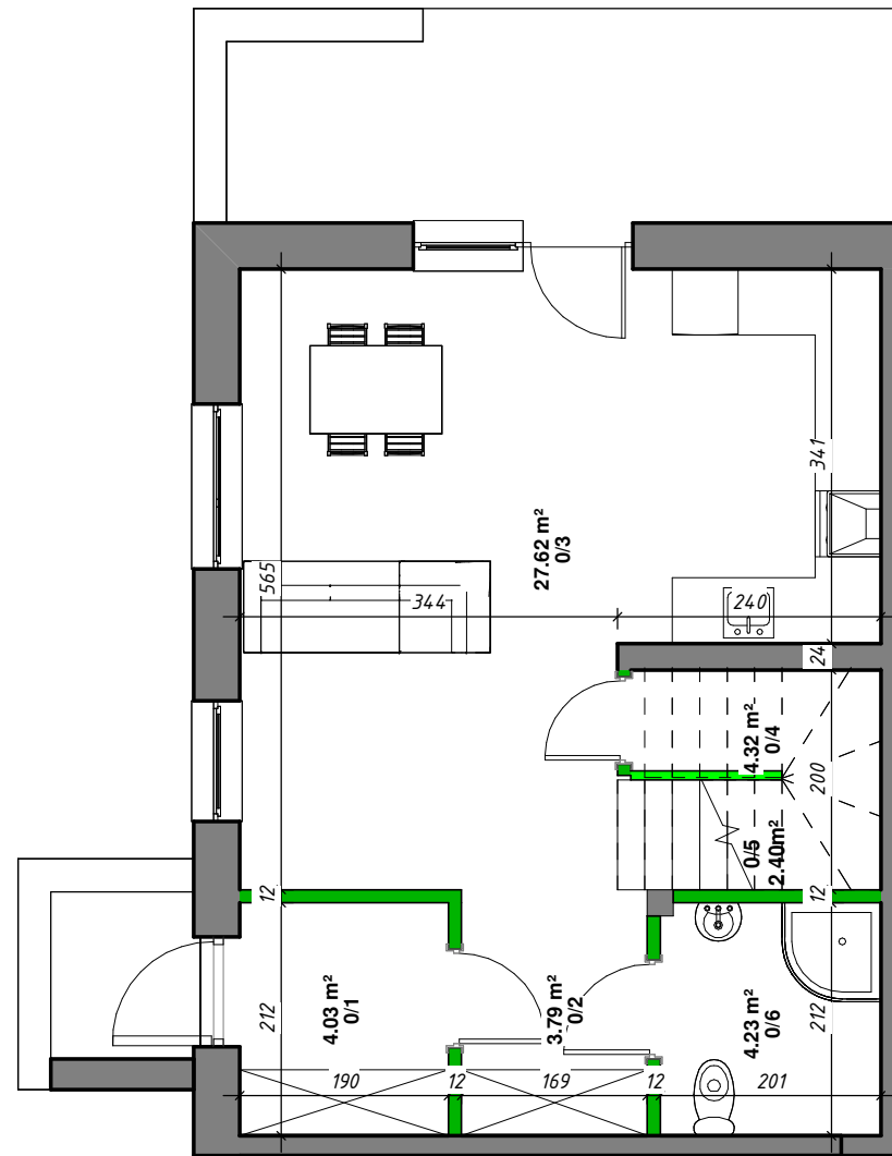
Rzut parteru
