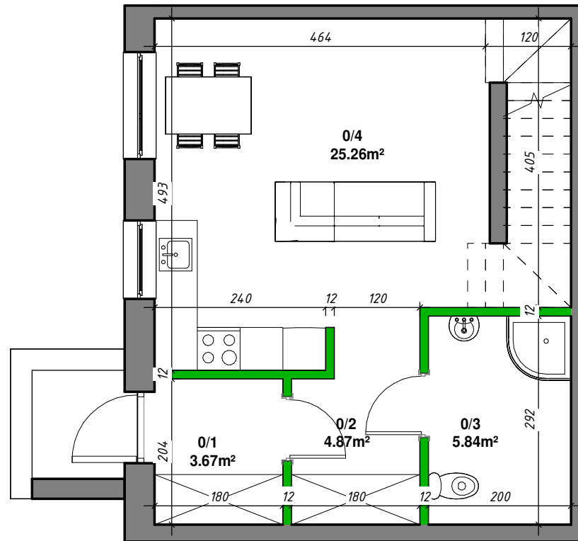
Rzut parteru
